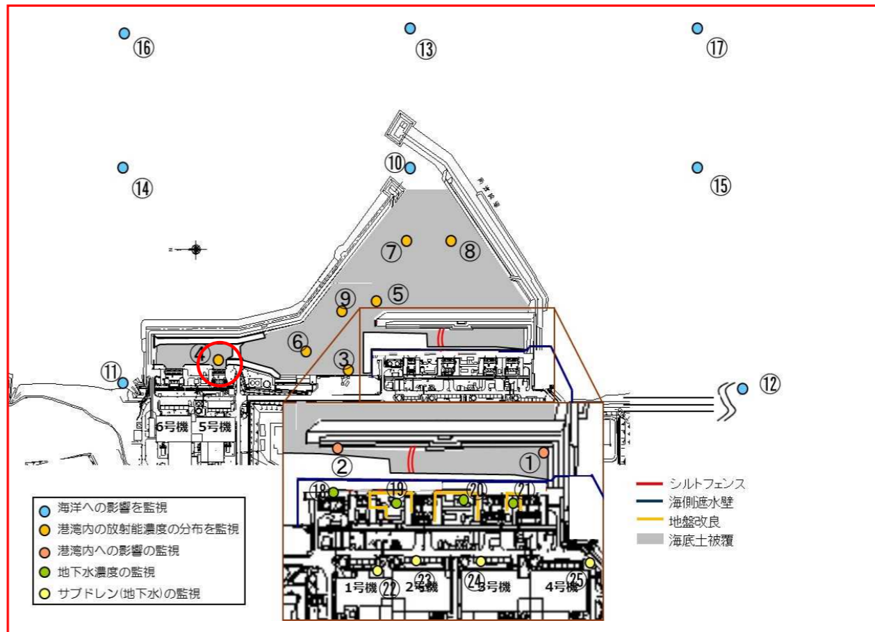
図2 港湾内外海水及び地下水のモニタリング計画 (サンプリング箇所)
