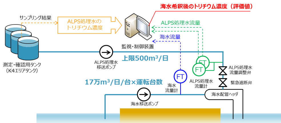
図-9 海水希釈後のトリチウム濃度の評価式
