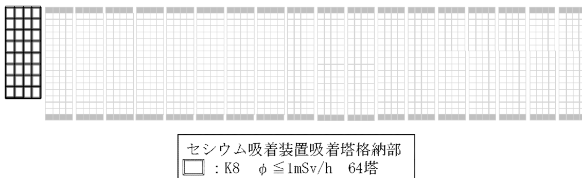
図2 第三施設の吸着塔格納配置計画 (φ：吸着塔側面線量率) (セシウム吸着装置吸着塔格納部：黒線部)
