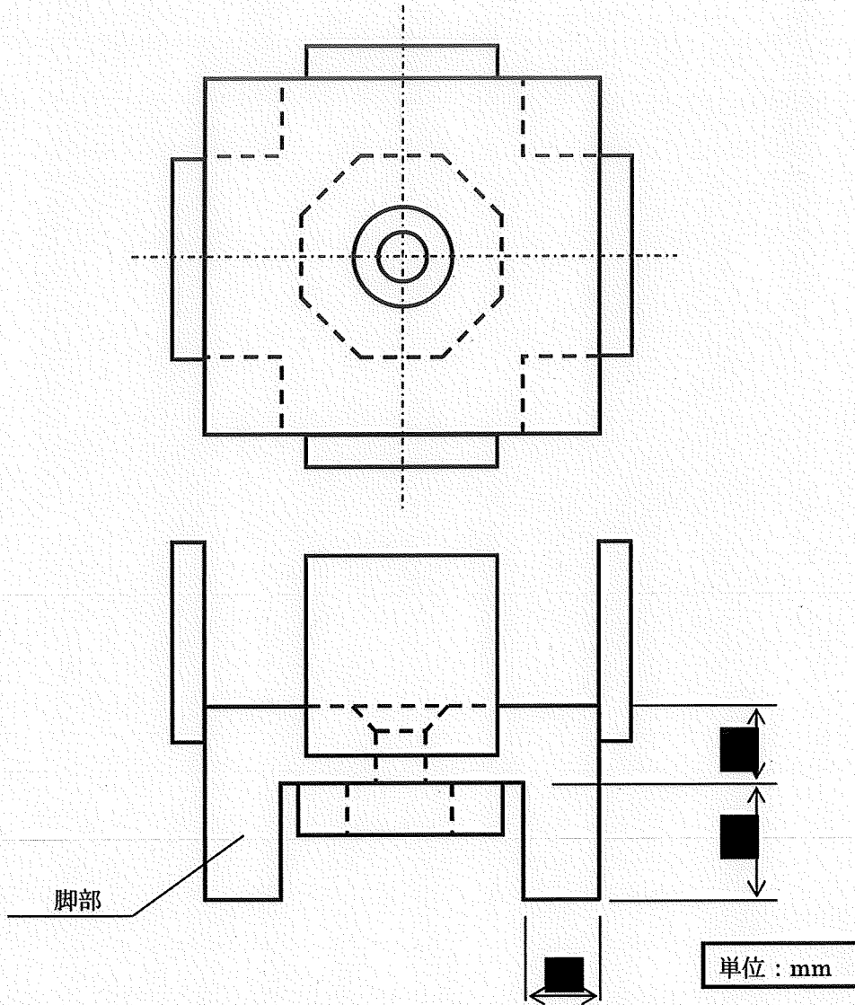
図-6 大口格子用ツールの応力評価箇所
