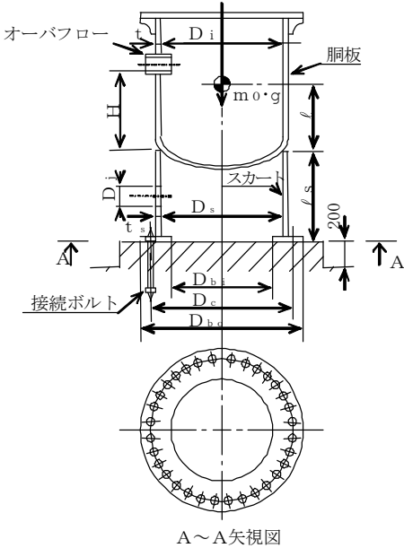
A ~ A 矢視図
