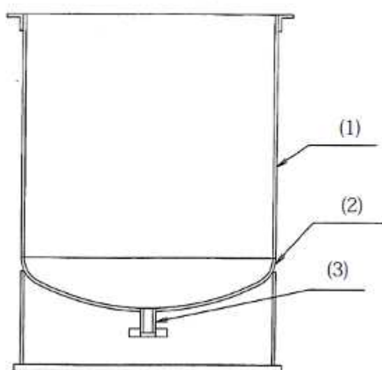
図－１－１ 処理水受入タンク 概要図
