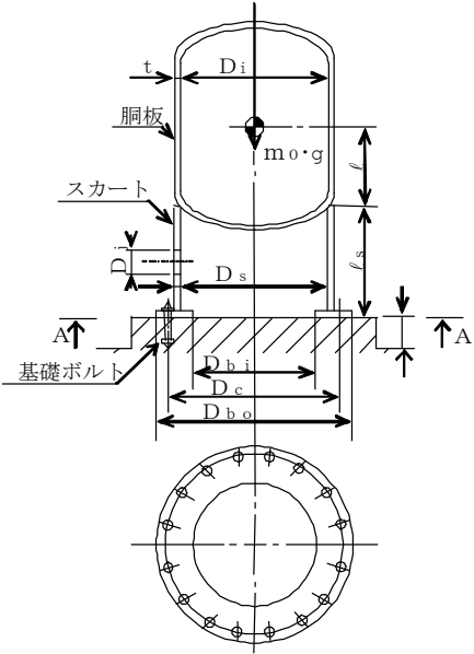
A～A矢視図
