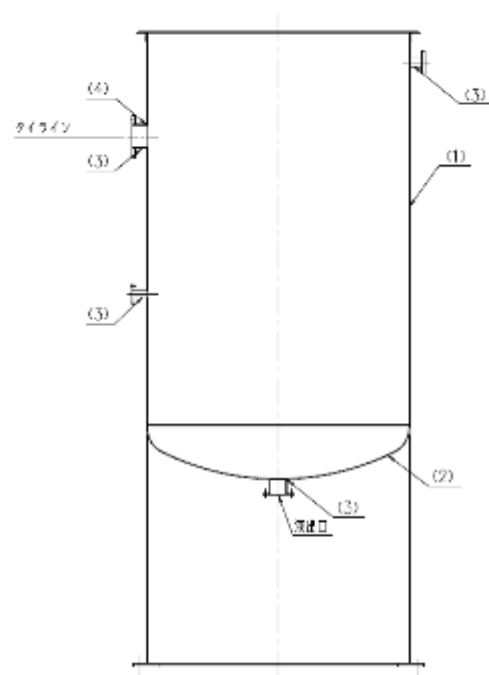
図－１－２ 共沈タンク，供給タンク 概要図
