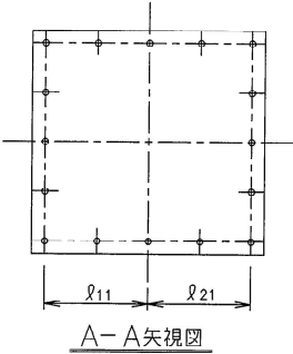
A-A矢視図
