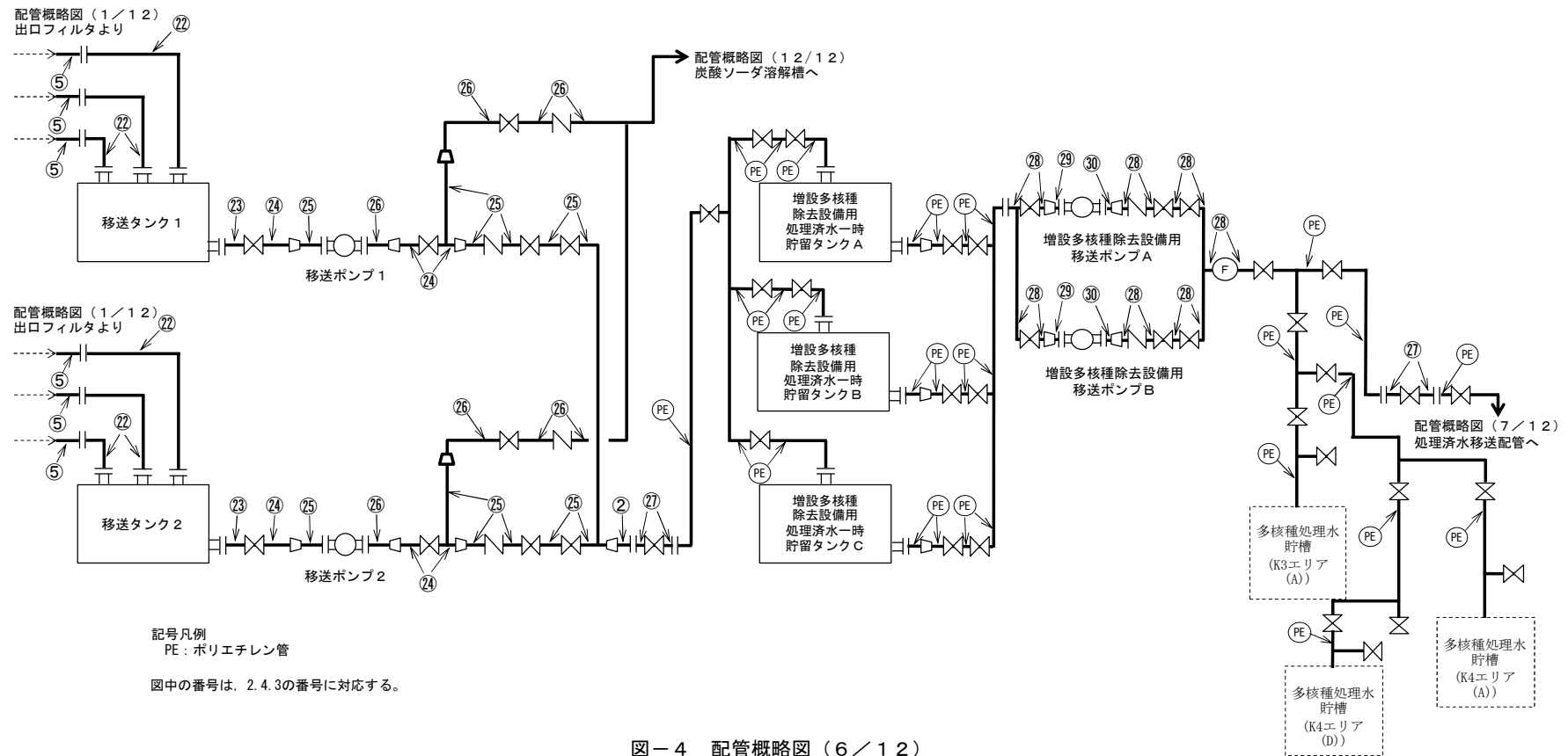
図ー 4 配管概略図 (6 / 1 2)
