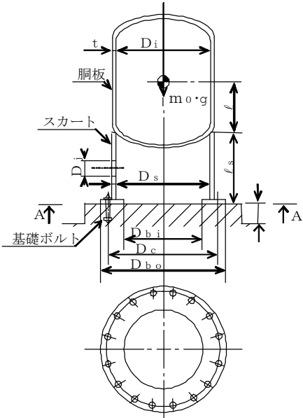
A～A矢視図
