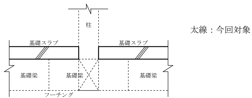
図－4 基礎スラブと柱・基礎梁の模式図
