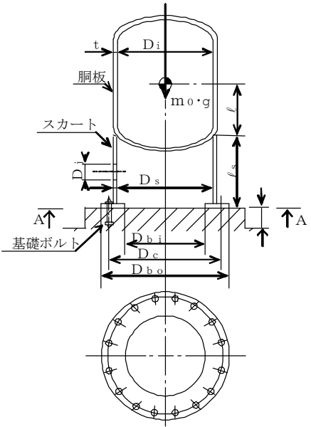
A～A 矢視図
