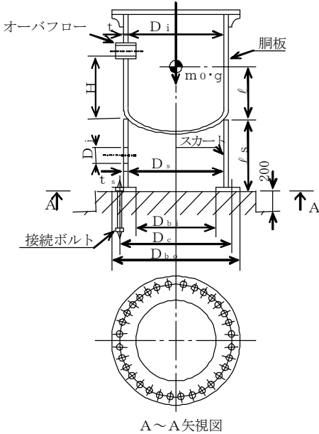
A～A矢視図
