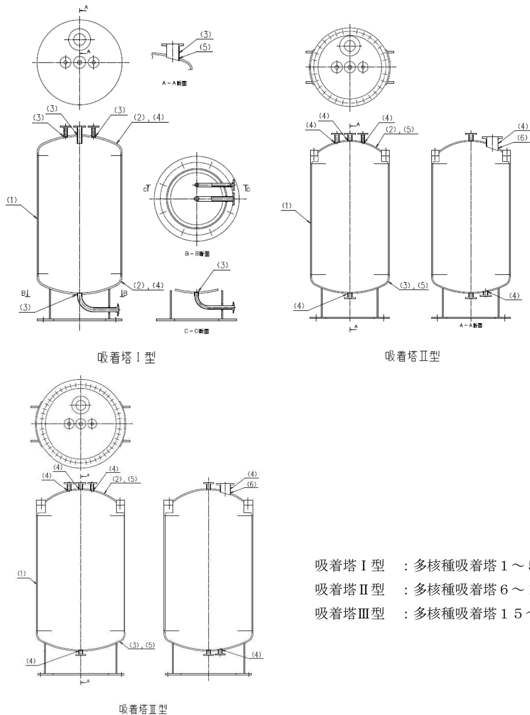
図－2 吸着塔 概要図
