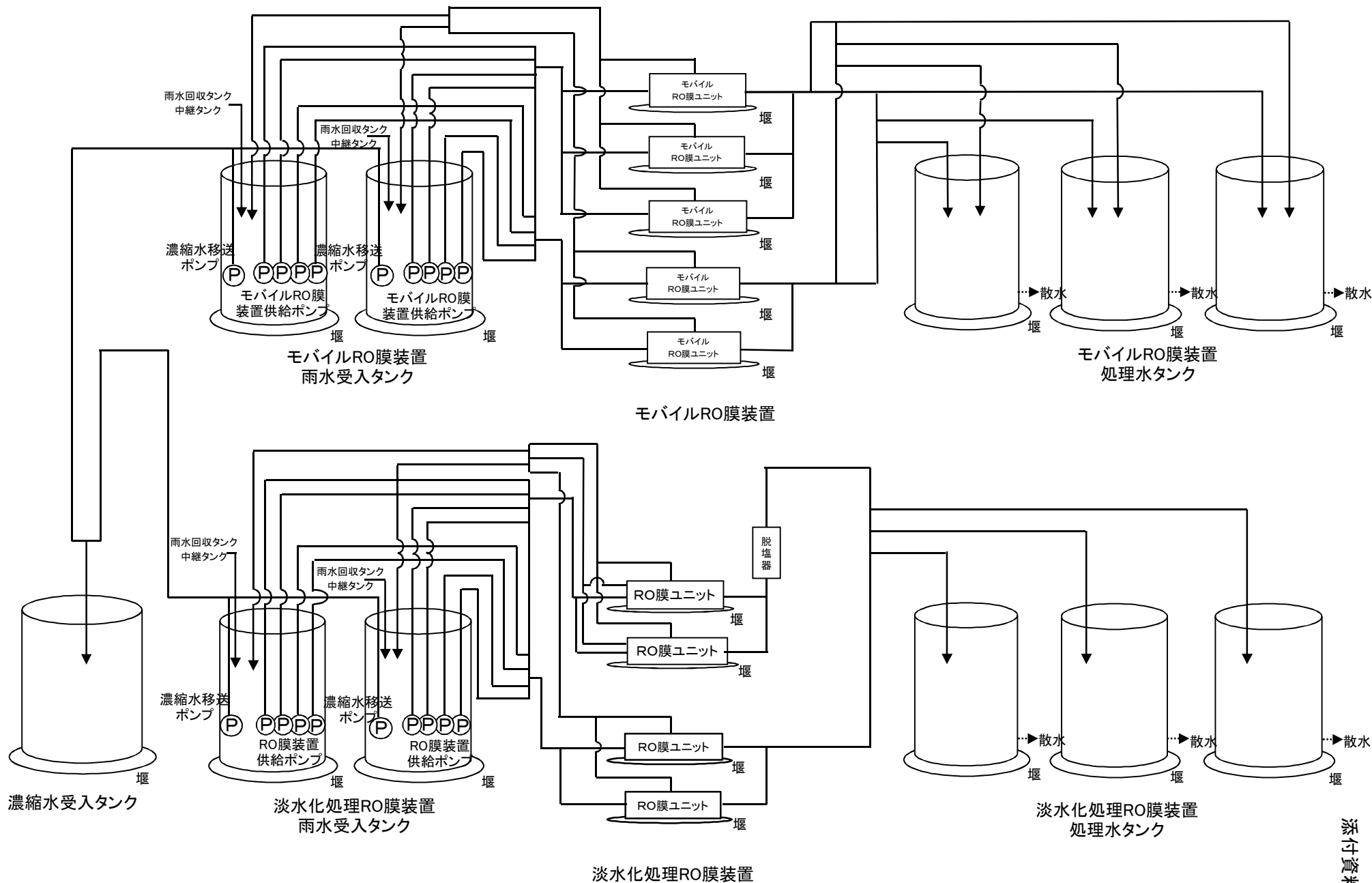
全体概略図(1/2)
