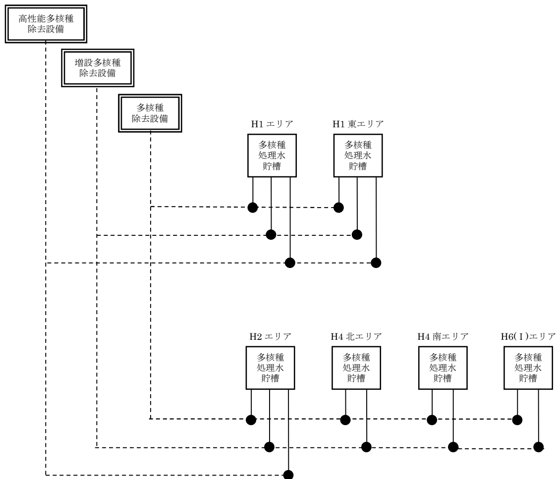
移送配管系統図 (H1, H1 東, H2, H4 北, H4 南, H6(I))
