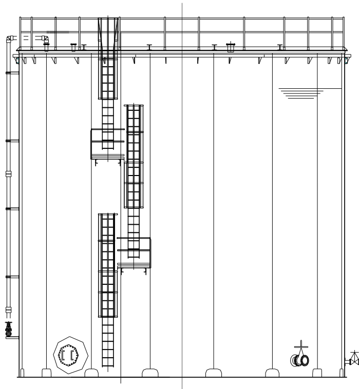
溶接型タンク概略図 (J6, K1 北, J7, H6(I))
