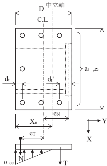
基礎ボルトの引張応力計算モデル (i) e_r < -(D/6 + d_t'/3) ・基礎ボルトに引張応力発生
