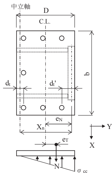
基礎ボルトの引張応力計算モデル (iv) D/6 \leq e_r < D/6 + d_t'/3 ・基礎ボルトに引張応力発生なし
