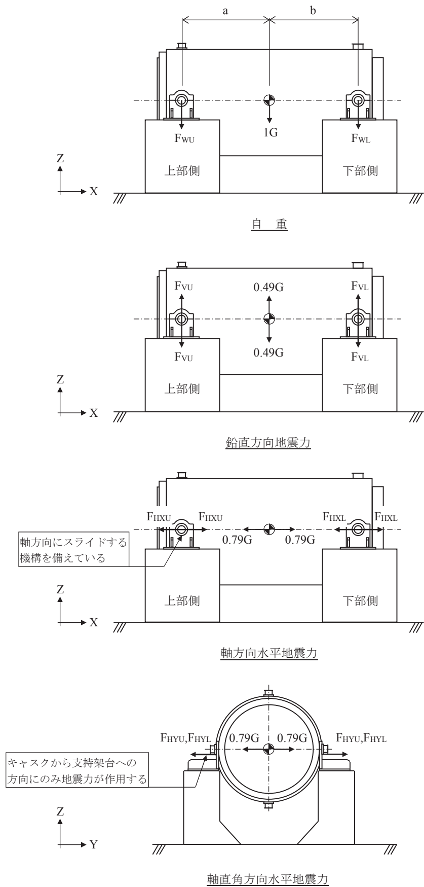
図3 鋼製支持架台に作用する荷重
