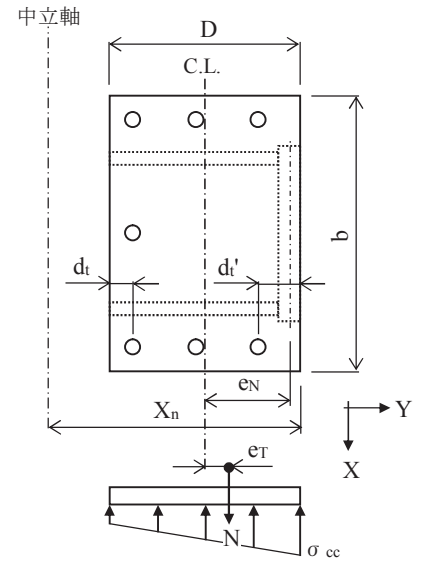
基礎ボルトの引張応力計算モデル (iii) -D/6 \leq e_r < D/6 ・基礎ボルトに引張応力発生なし
