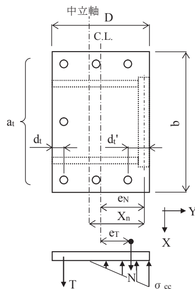
基礎ボルトの引張応力計算モデル (v) D/6 + d_t'/3 \leq e_r ・基礎ボルトに引張応力発生
