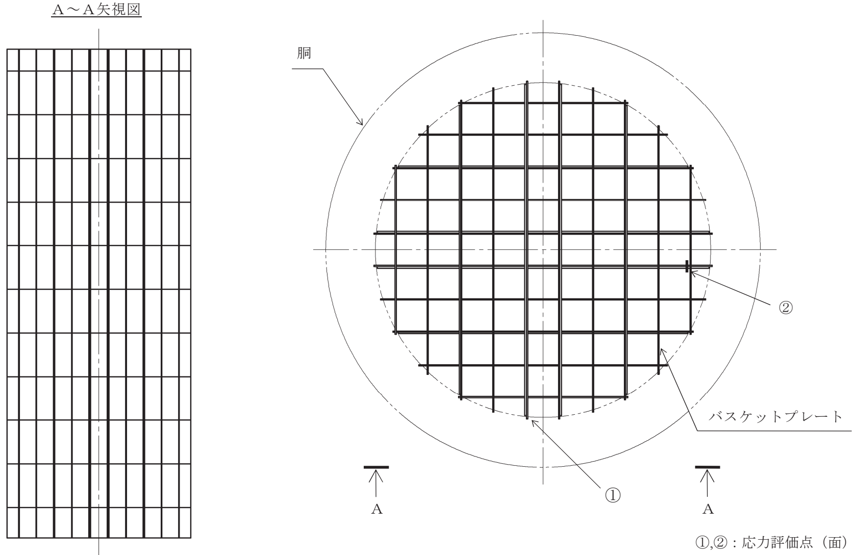
図2 バスケットの応力解析箇所
