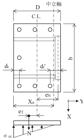
基礎ボルトの引張応力計算モデル (ii) -(D/6 + d_t'/3) \leq e_r < -D/6 ・基礎ボルトに引張応力発生なし
