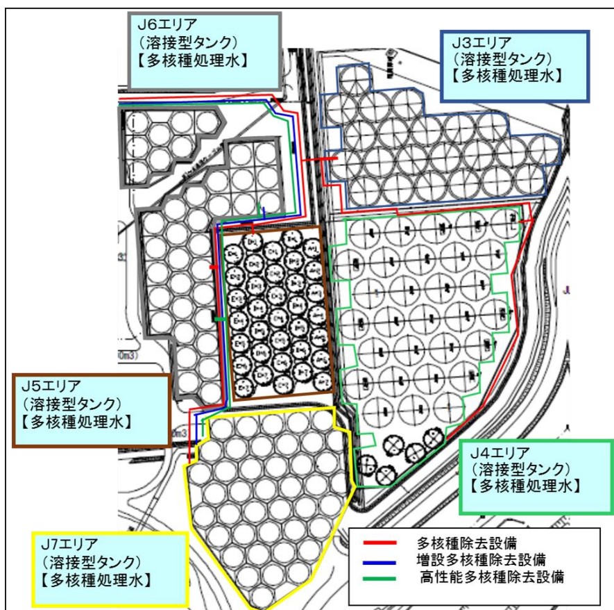
タンクエリア詳細図
