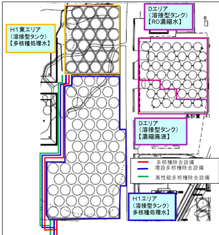
タンクエリア詳細図
