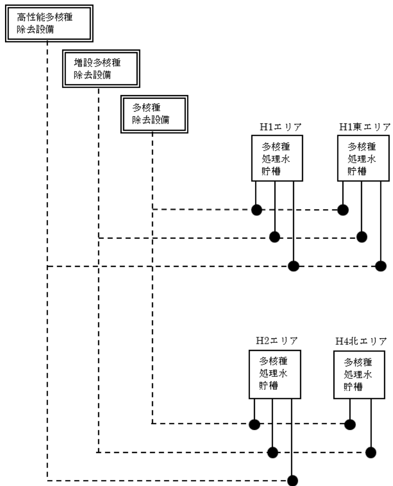
移送配管系統図 (H1, H1 東, H2, H4 北)
