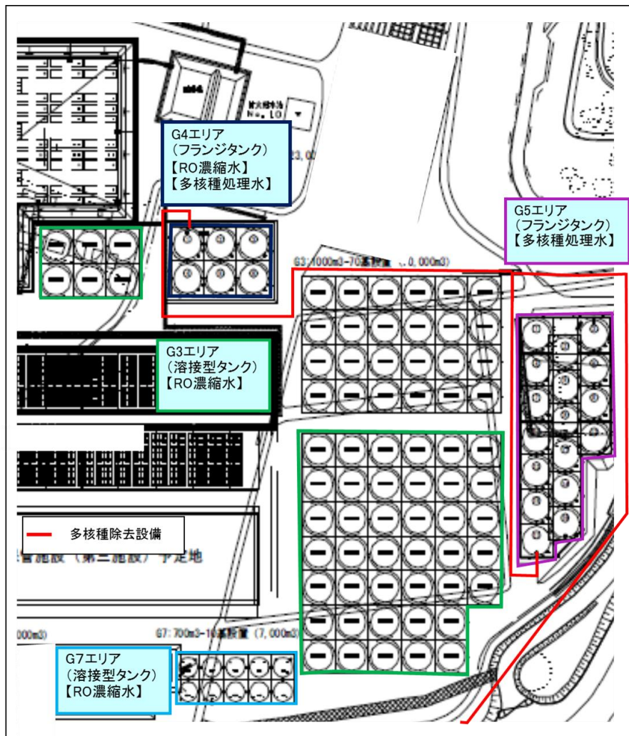
タンクエリア詳細図
