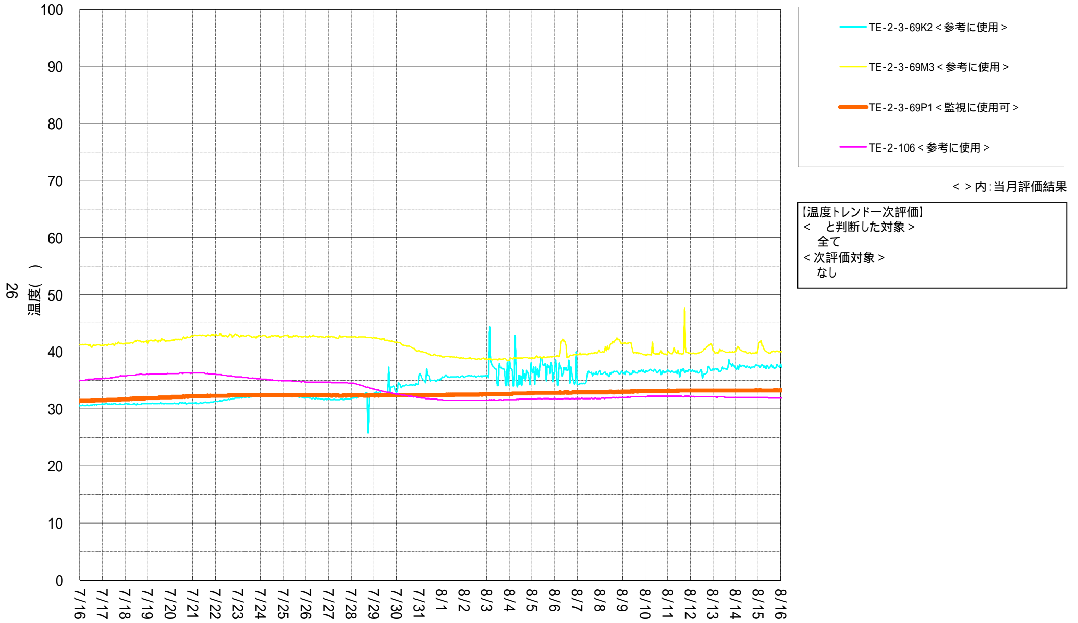
2号機 RPV周辺温度計(下部)
