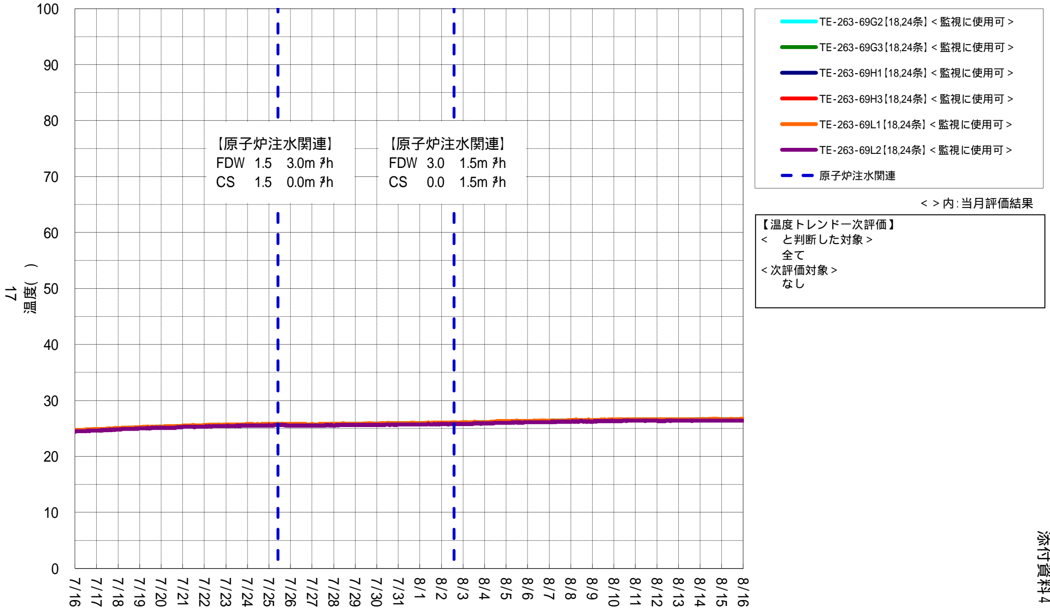
1号機 実施計画関連温度計 (RPV)
