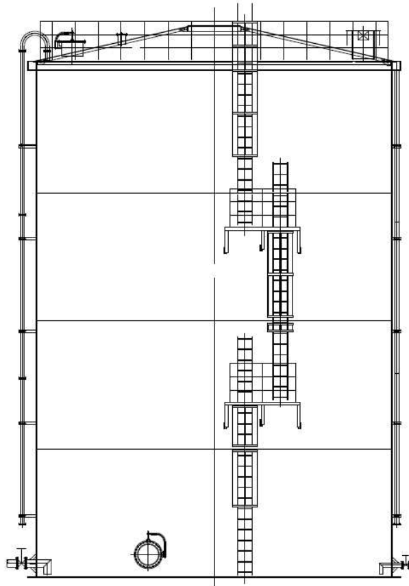
溶接型タンク概略図 (D, K2, K4, H4 南(1, 140m 3 ))
