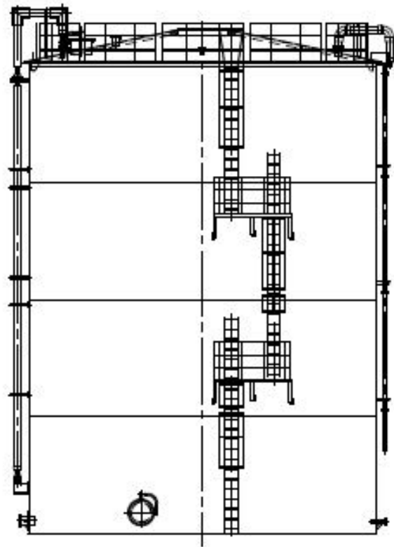
溶接型タンク (H4 南(1, 140m 3 ))
