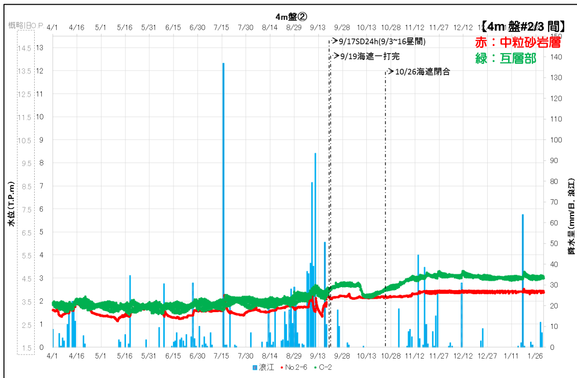
図一8. 1 2 中粒砂岩層／互層部，細粒・粗粒砂岩の水頭比較（4 m盤②）
