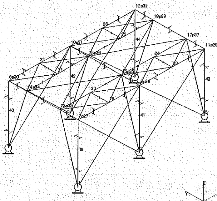
図一五 ディスクフィルタ解析モデル
