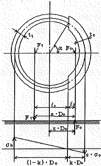
基礎の荷重説明図
