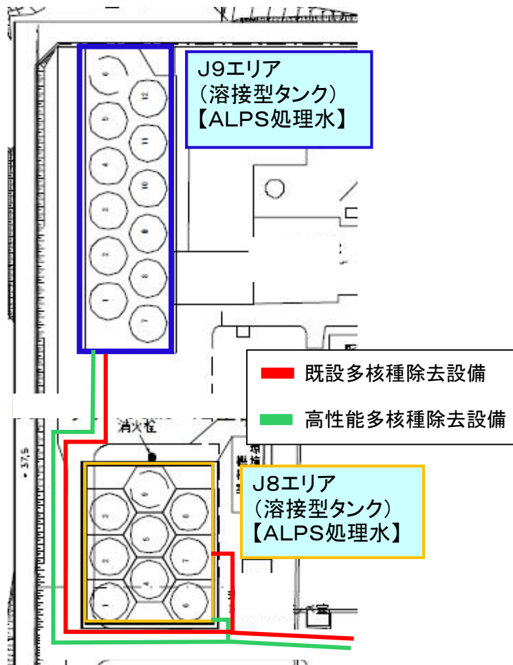
タンクエリア詳細図
