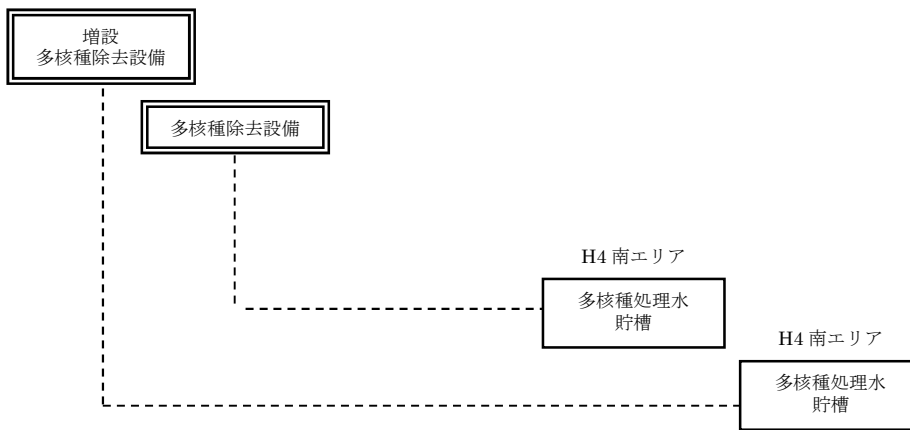
移送配管系統図（H4 南）
