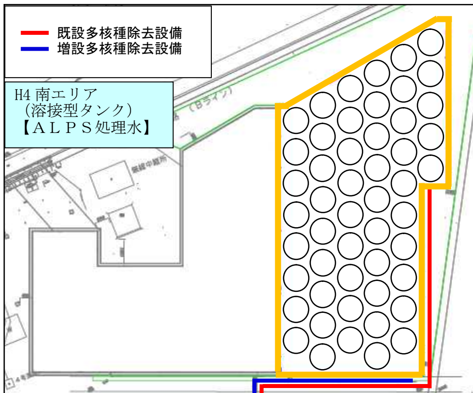
タンクエリア詳細図
