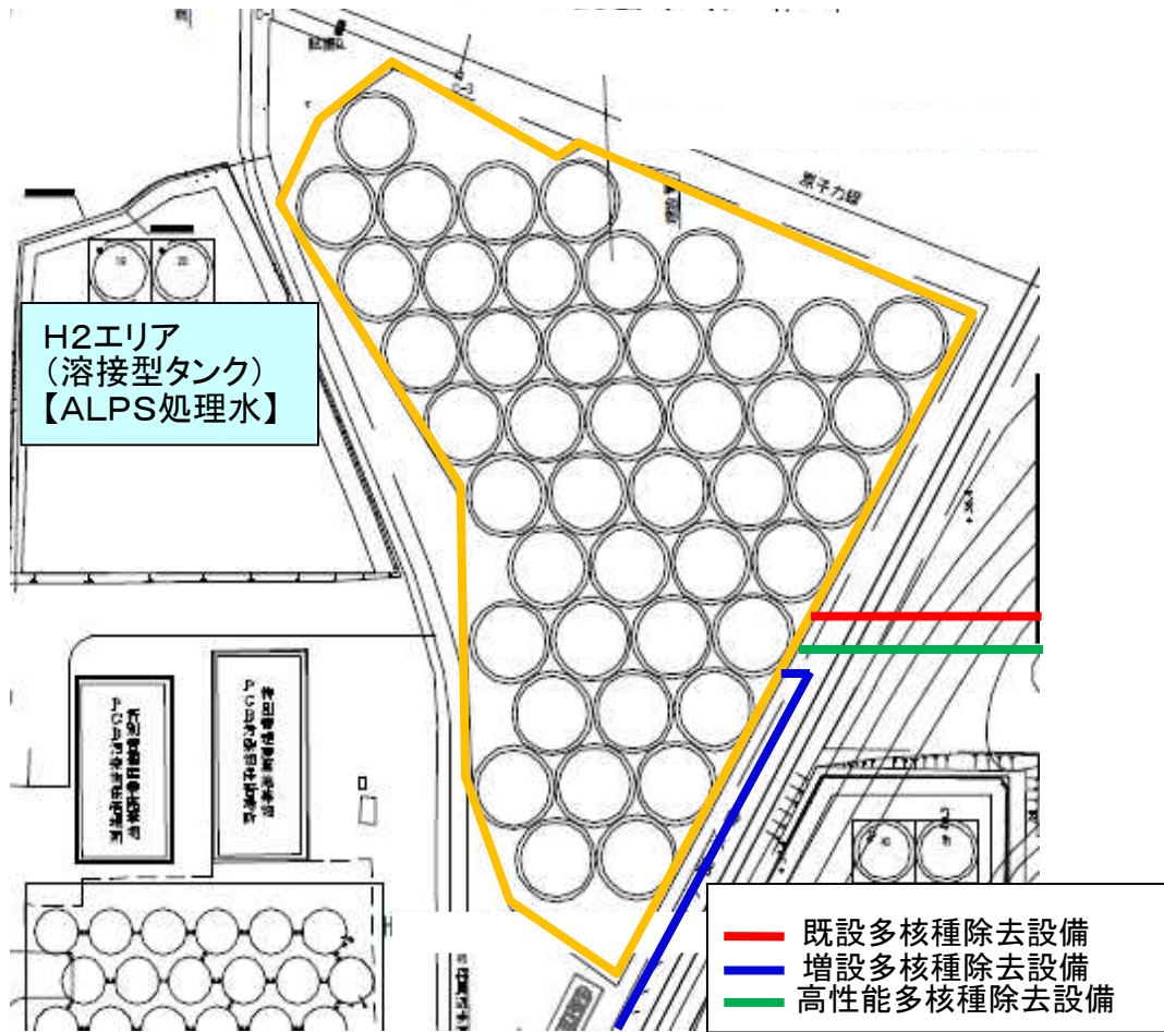
タンクエリア詳細図
