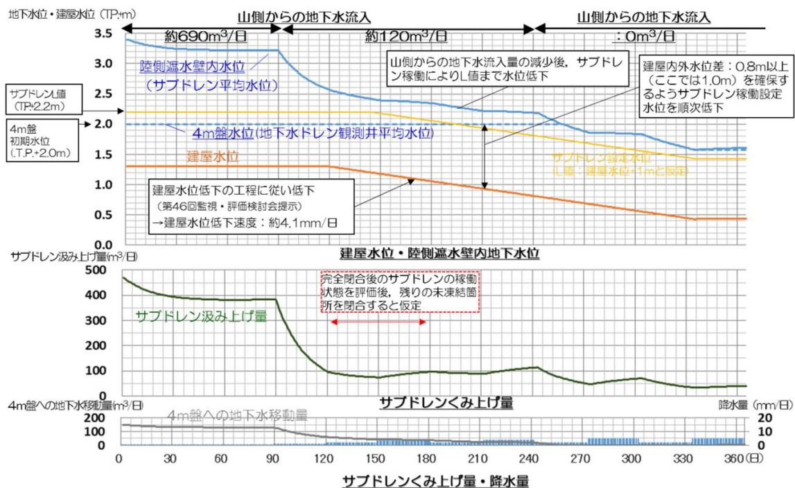
図－6 一部閉合（Ⅱ）後の建屋周辺における地下水位変動の想定
