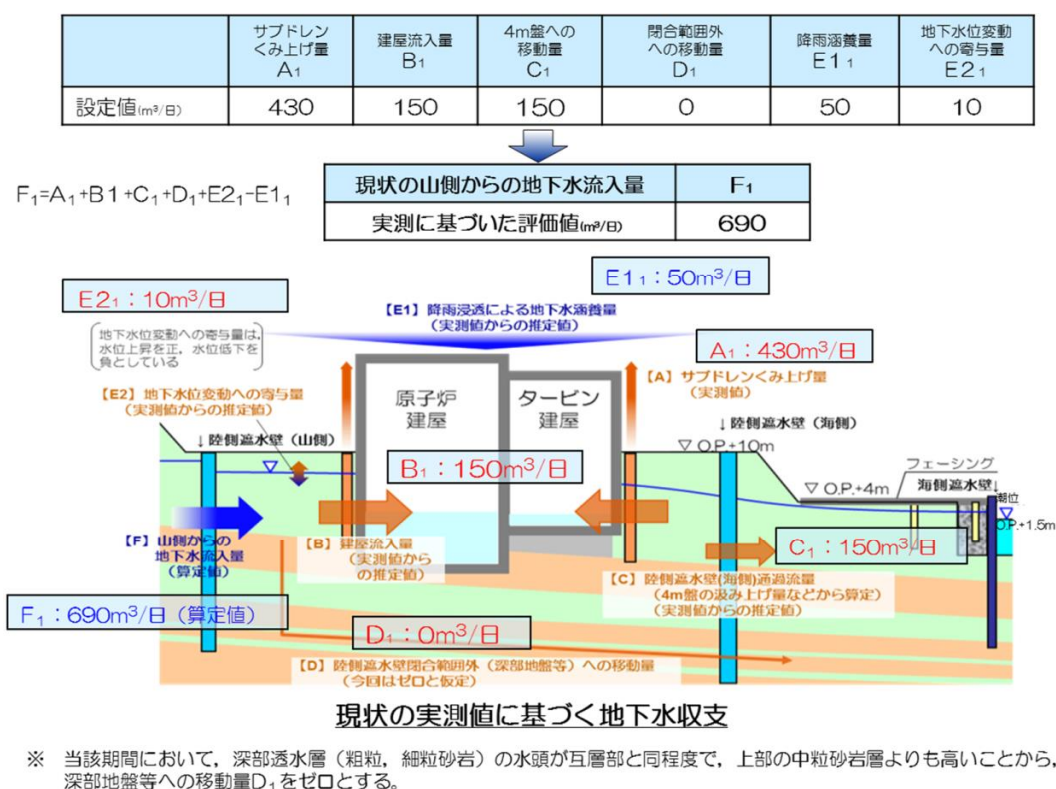
図－2 一部閉合（Ⅱ）前の山側からの地下水流入量の想定
