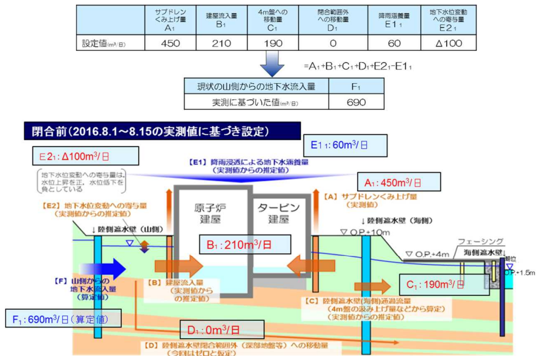
図-3 一部閉合前の山側からの地下水流入量の想定
