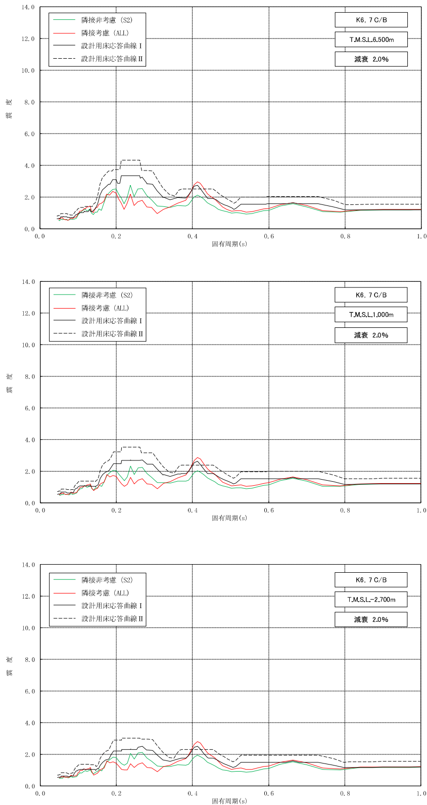
図添 1-2 床応答スペクトルの比較（コントロール建屋，水平方向，減衰 2.0%）（2/2） 別紙 4-14
