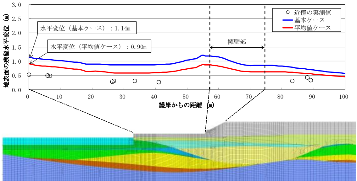
図 3-12 護岸からの距離と地表面水平変位の関係 (南断面)
