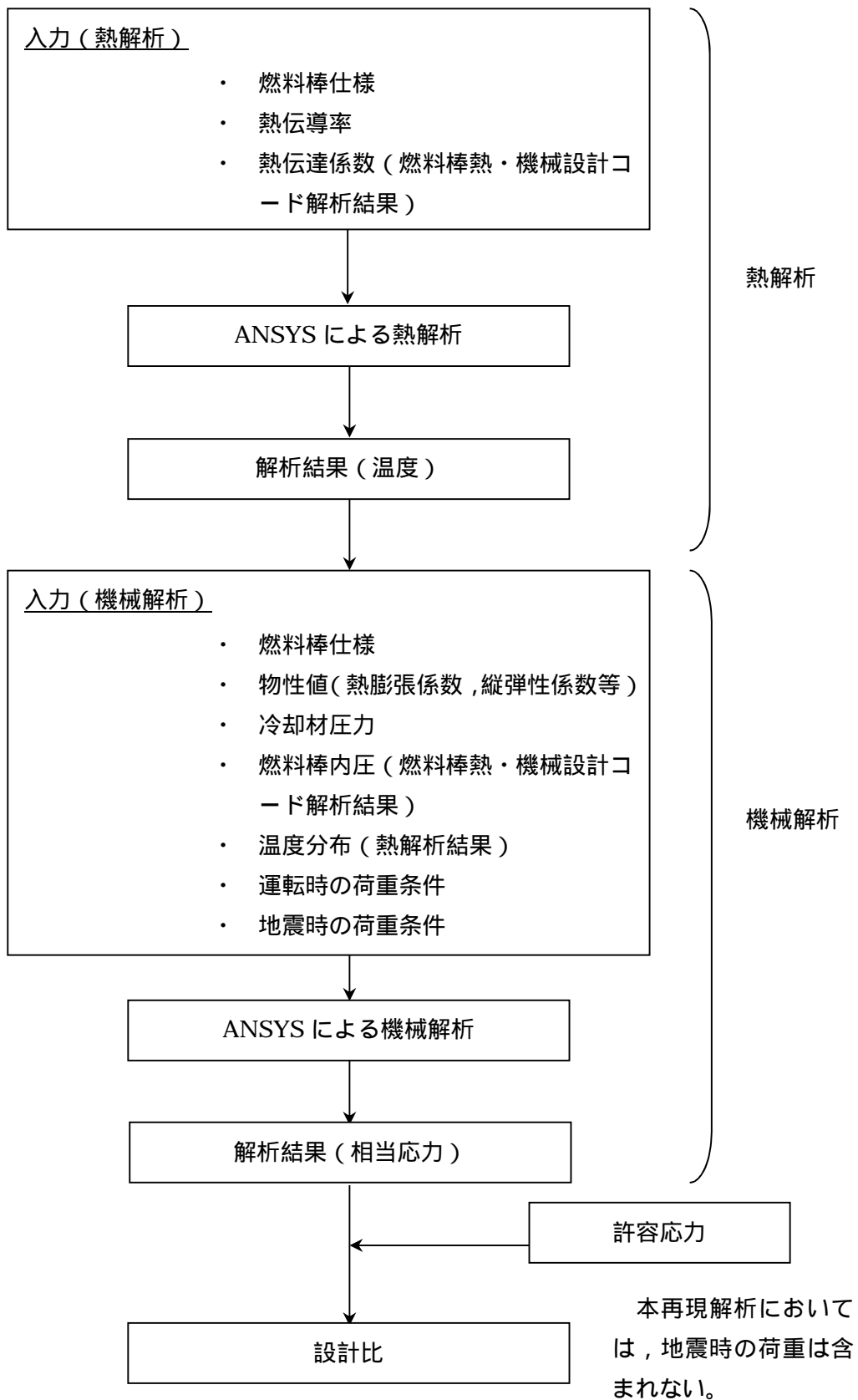
添付7-1図 下部端栓溶接部の応力評価のフロー
