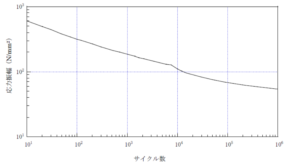
ジルカロイの設計疲労曲線*)
