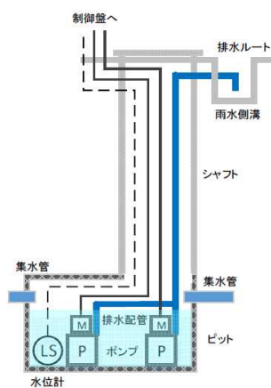
第 2-2 図 サブドレン設備の概略図
