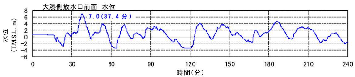
第 2.1.1-1(b) 図 入力津波の波形 (大湊側放水口前面)
