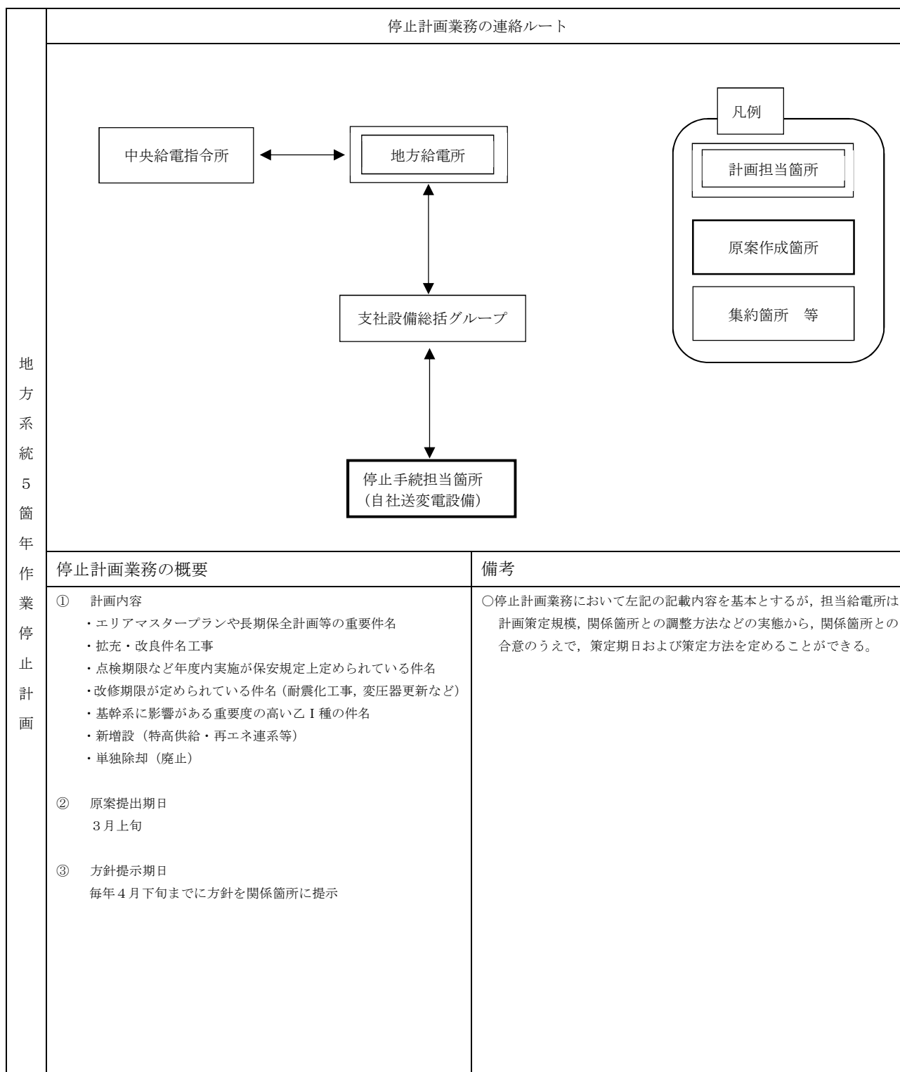
図 8 - 3 作業停止計画業務の概要(地方系統 5 箇年作業停止計画)
