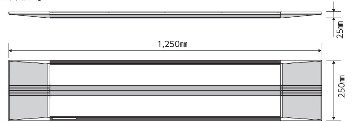
照明器具外形図
