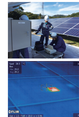
発電所メンテナンス ホットスポット例(左下)、ドローンによる点検(右)
