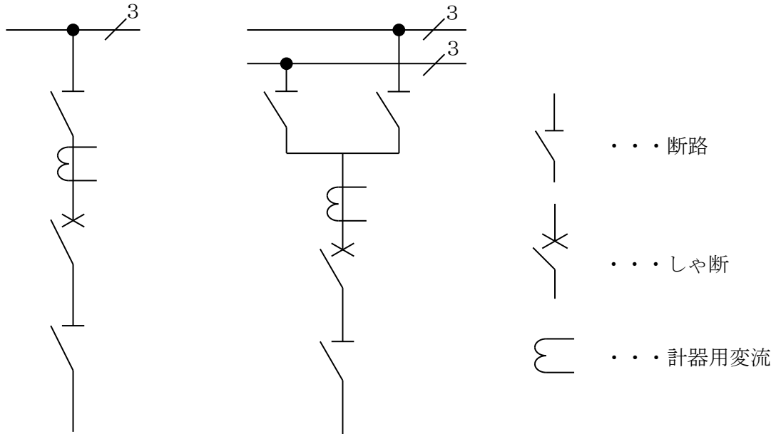
単母線の場合
