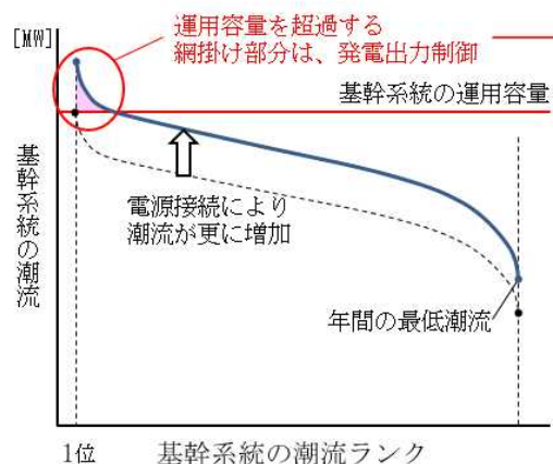
【想定潮流（イメージ）】
