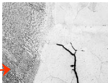
図8-2 観察位置D(観察倍率: ×100) 0.1mm
