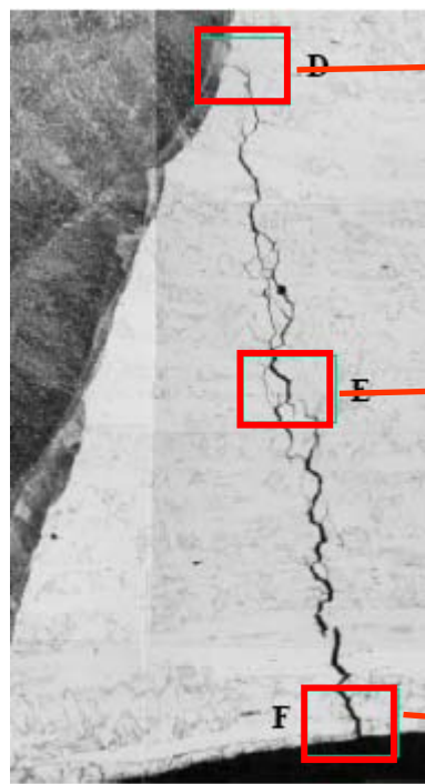
図8-1 ひび全体 (観察倍率: ×25)
