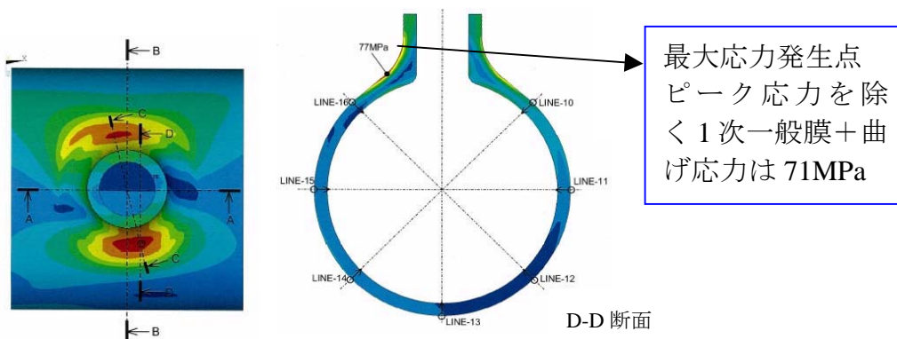
図 2-2 FEM 解析結果（応力コンター図）
