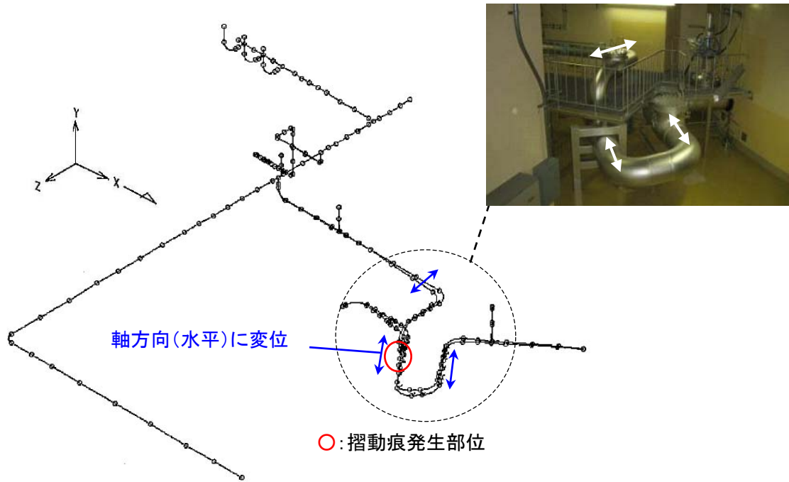
図4-3. モード図 (1次)
