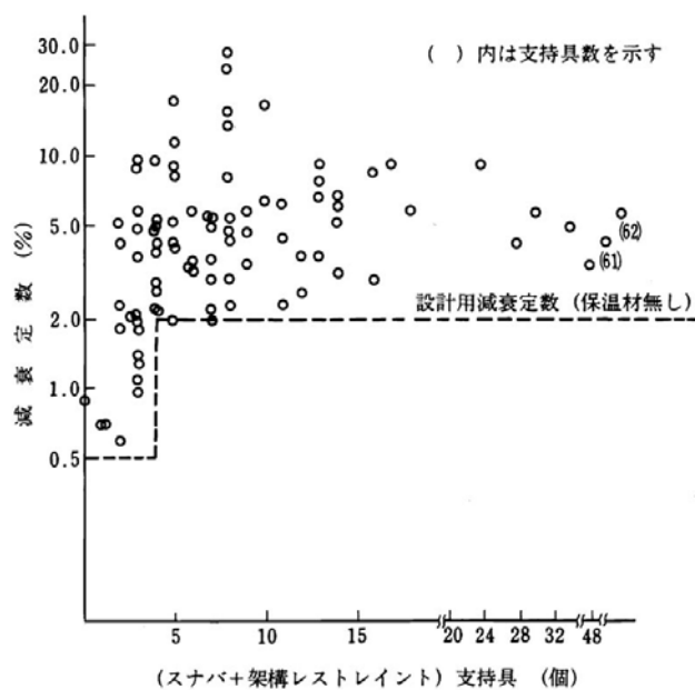
図4 減衰定数データ
