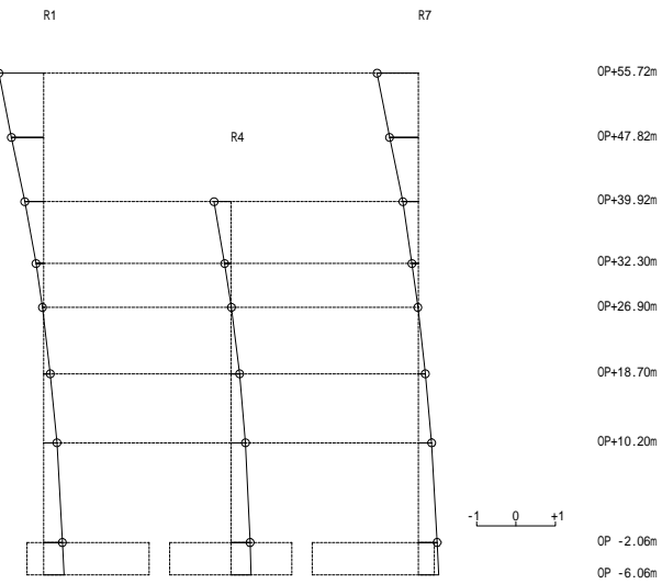
床柔モデル
