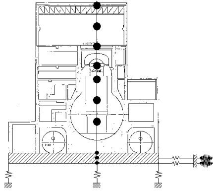
(工認設計時)
