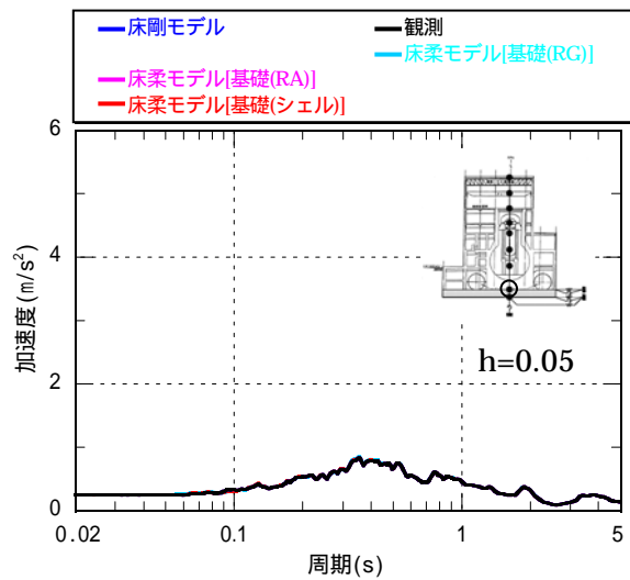
基礎版上 (O.P. -2.06m)
