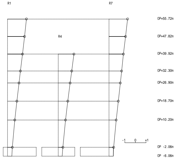
床柔モデル
