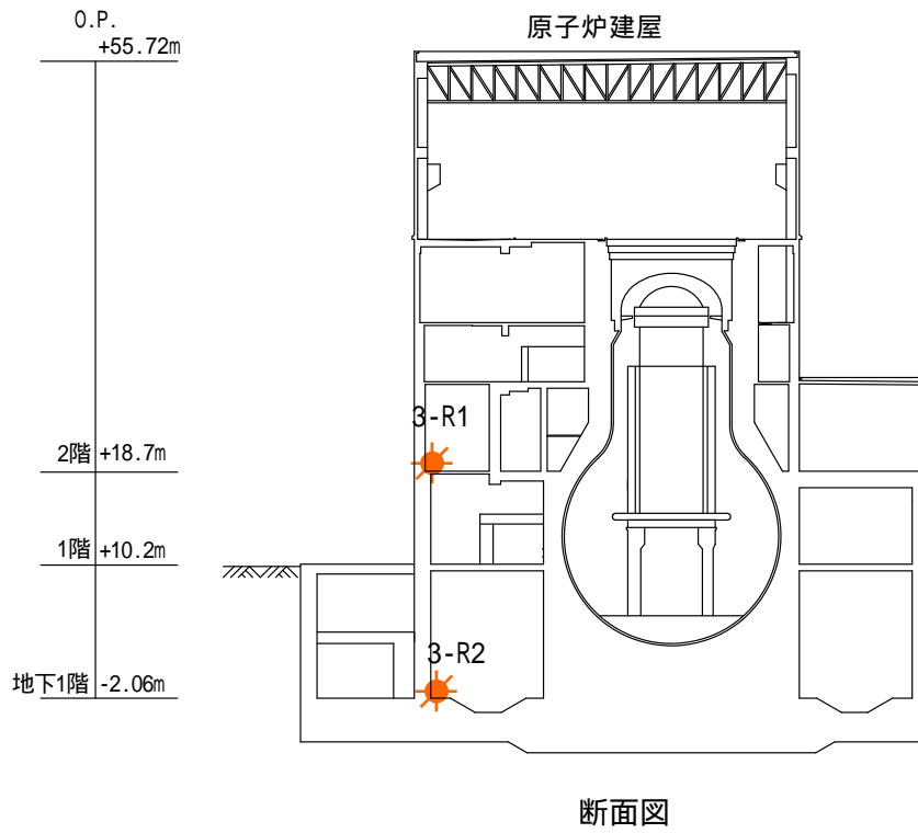
第3図 福島第一 3号機原子炉建屋 地震計配置図
