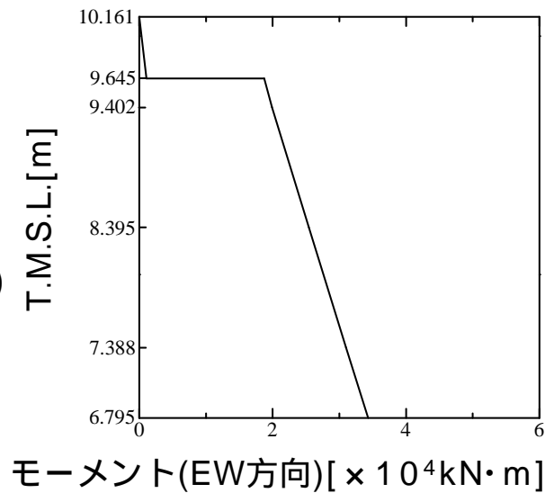
炉心シュラウド(下部胴)
