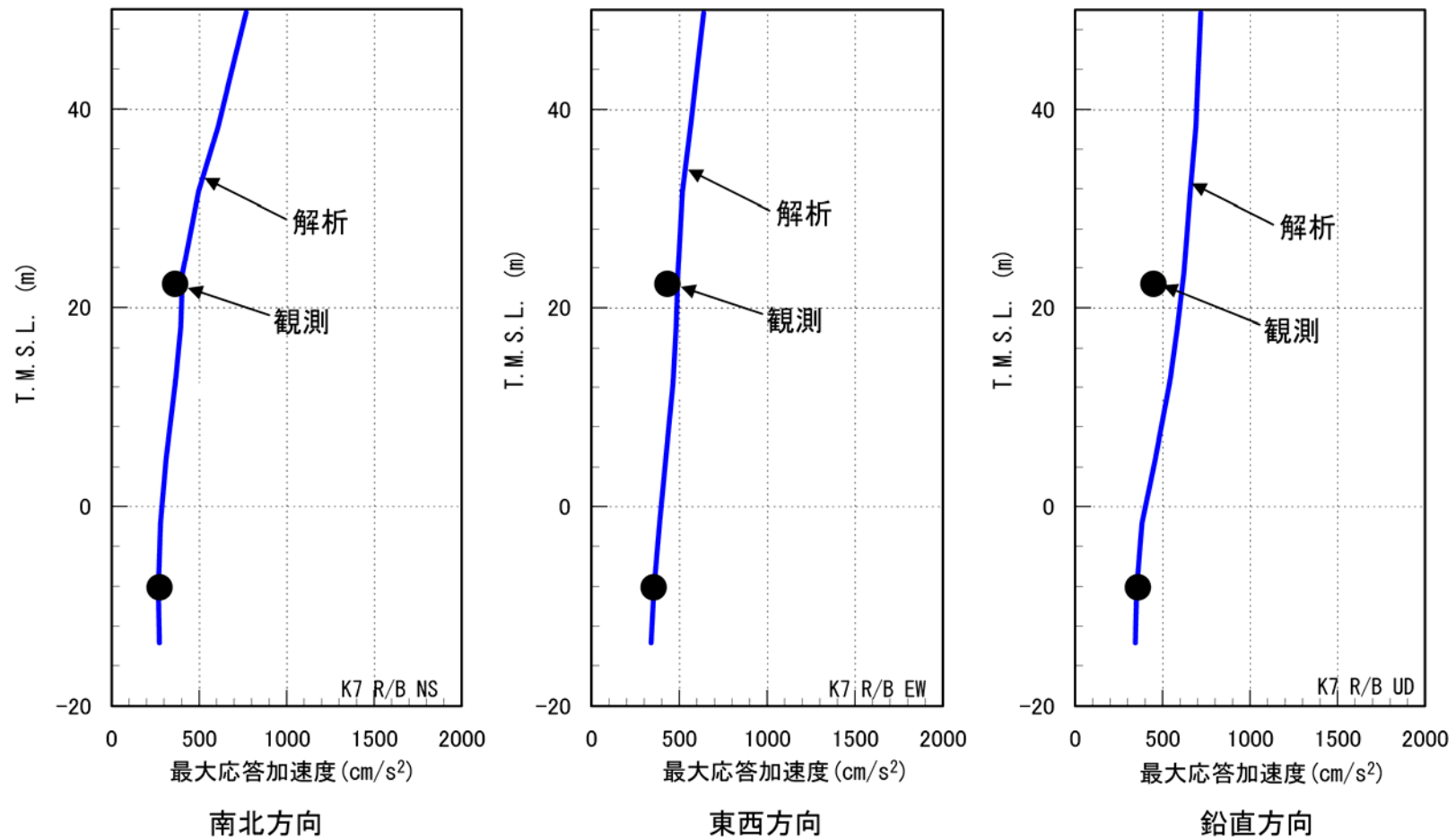
図-5.3.5 最大応答加速度の比較
