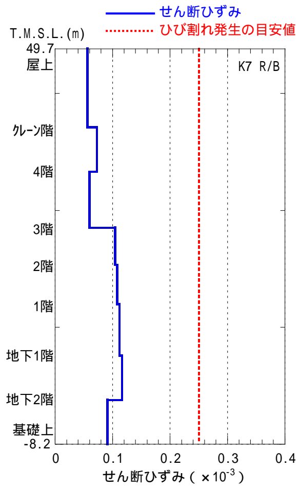
図-5.4.3 原子炉建屋 耐震壁のせん断ひずみ (南北方向)
