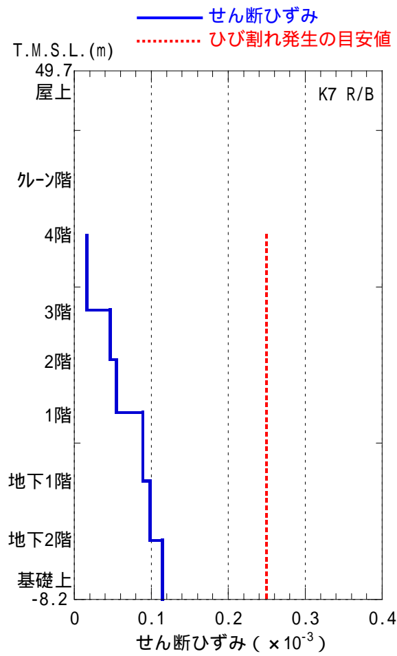
図-5.4.8 RCCVの鉄筋コンクリート部のせん断ひずみ(東西方向)
