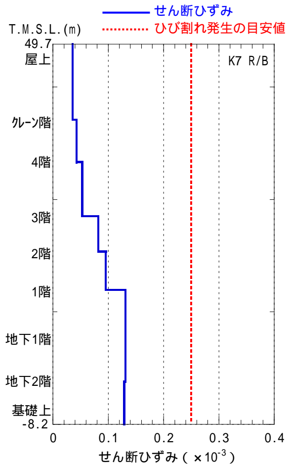
図-5.4.4 原子炉建屋 耐震壁のせん断ひずみ (東西方向)
