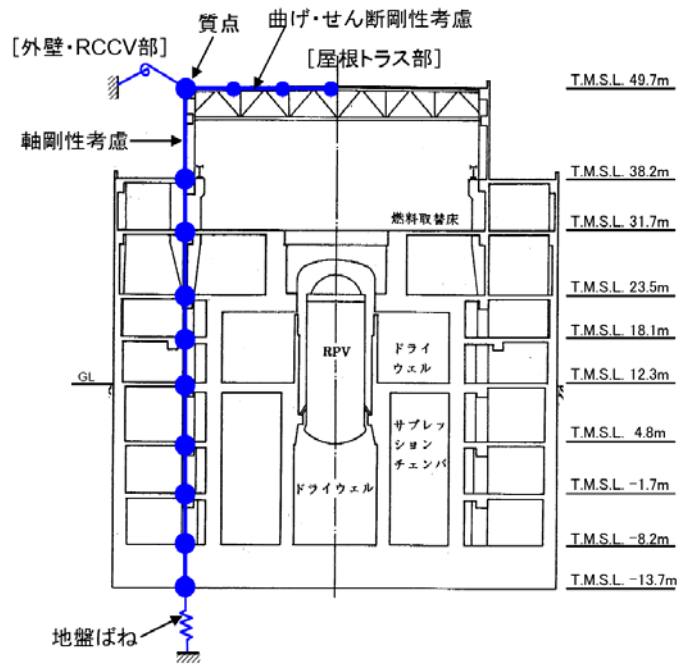
図-5.3.4 地震応答解析モデル（鉛直方向）
