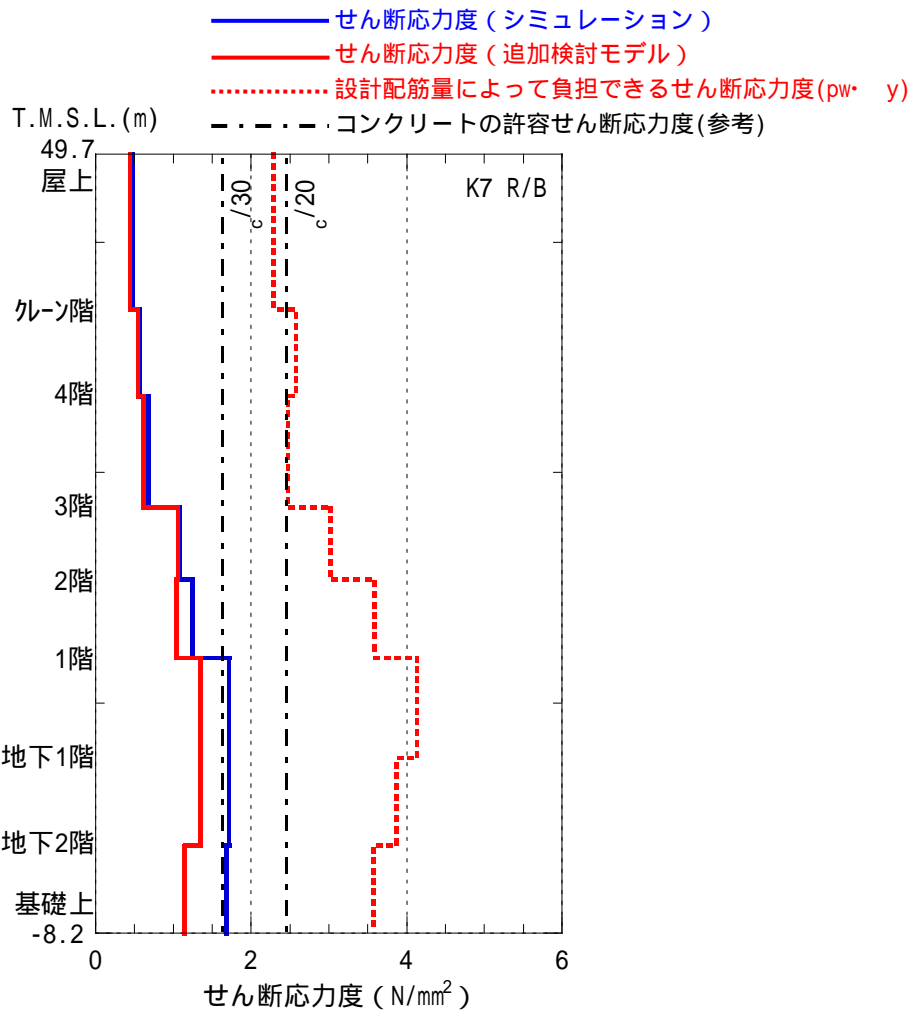
参図-7 原子炉建屋 耐震壁のせん断応力度 (東西方向)
