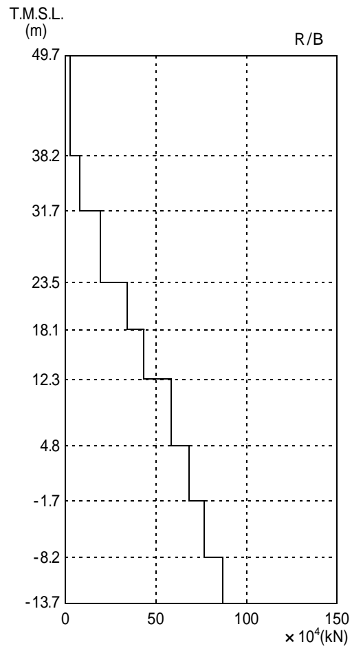
参図-8 最大応答軸力（鉛直方向）
