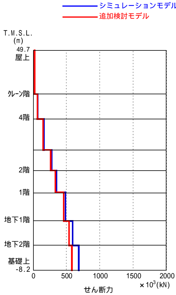
参図-15 原子炉建屋 最大応答せん断力（東西方向）
