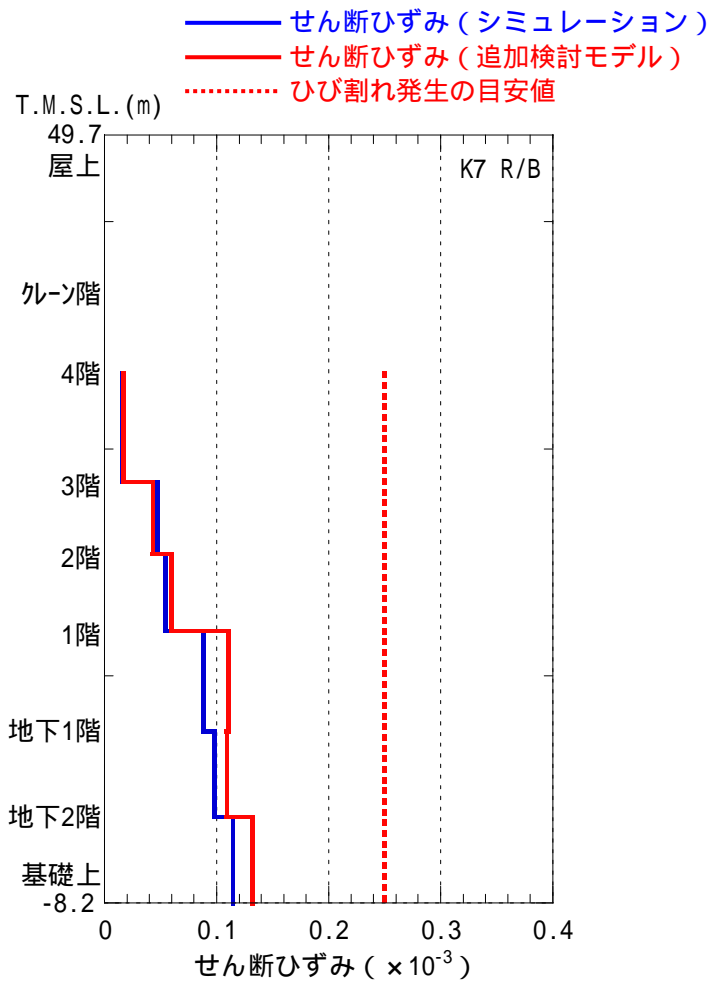
参図-13 RCCV の鉄筋コンクリート部のせん断ひずみ (東西方向)
