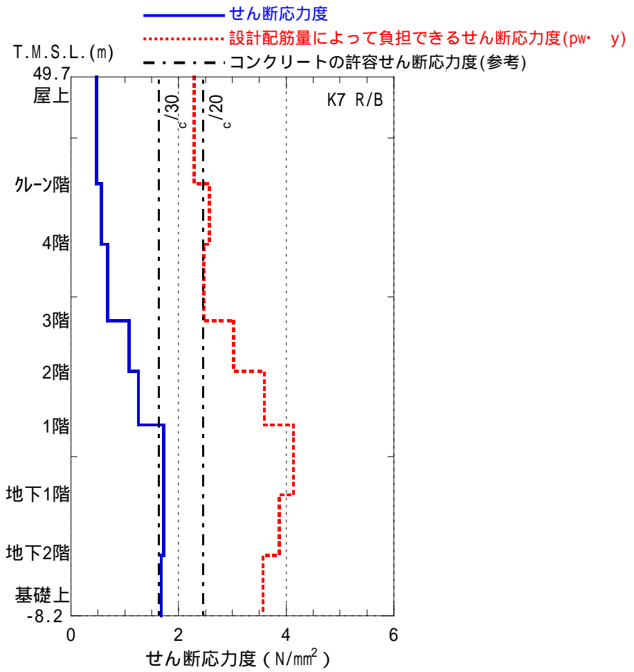
図-5.4.2 原子炉建屋 耐震壁のせん断応力度 (東西方向)
