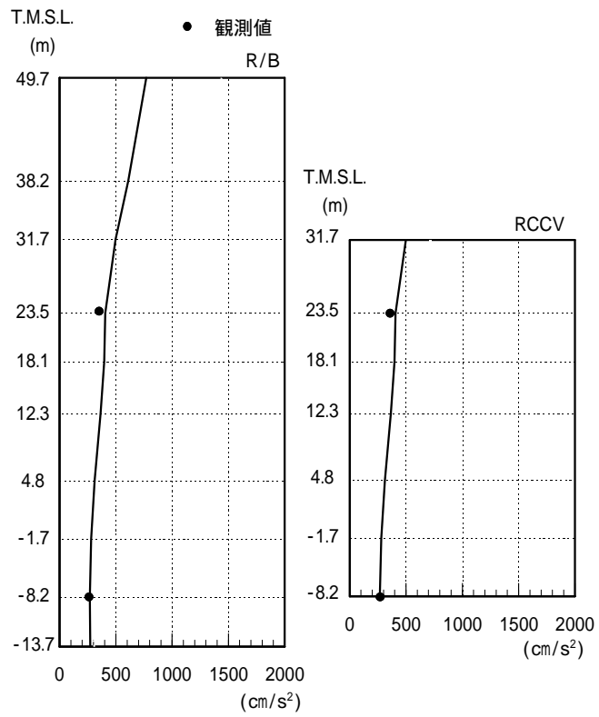
参図-1 最大応答加速度（南北方向）
