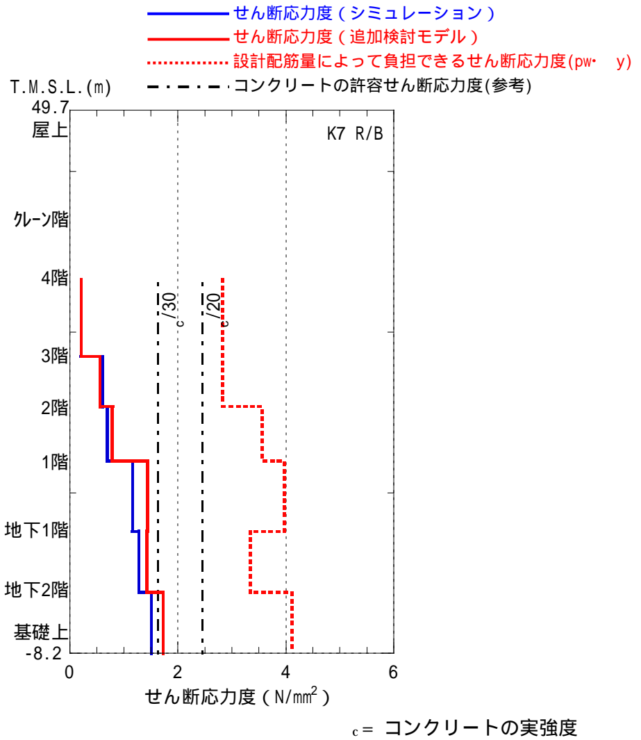
参図-11 RCCV の鉄筋コンクリート部のせん断応力度 (東西方向)
