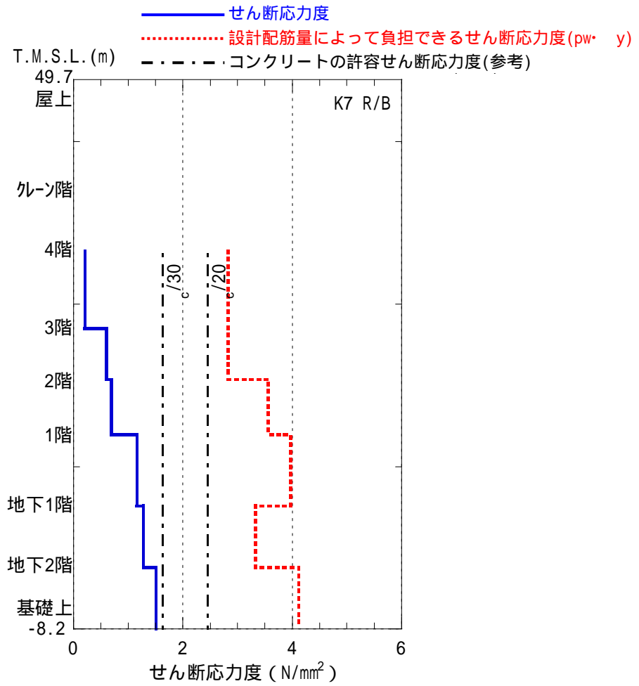
図-5.4.6 RCCVの鉄筋コンクリート部のせん断応力度(東西方向)
