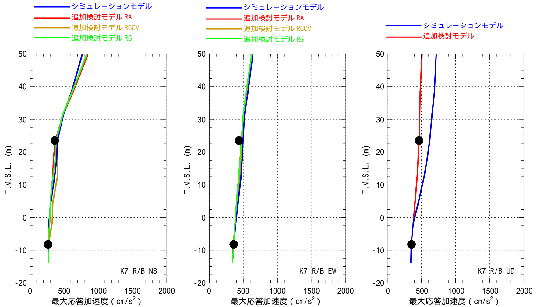
参図-2 最大応答加速度の比較
