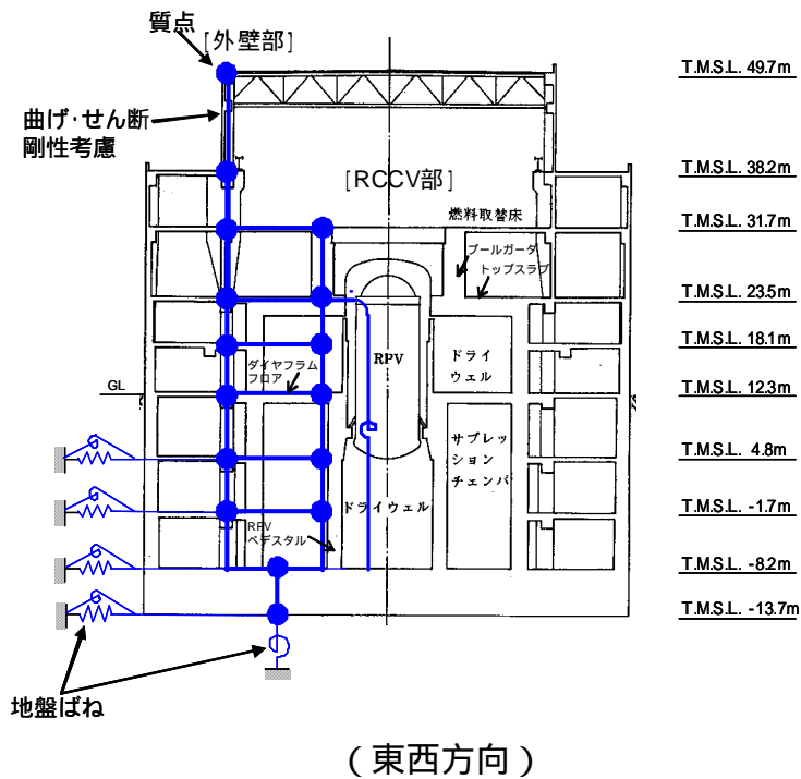
図-5.3.2 地震応答解析モデル (水平方向)
