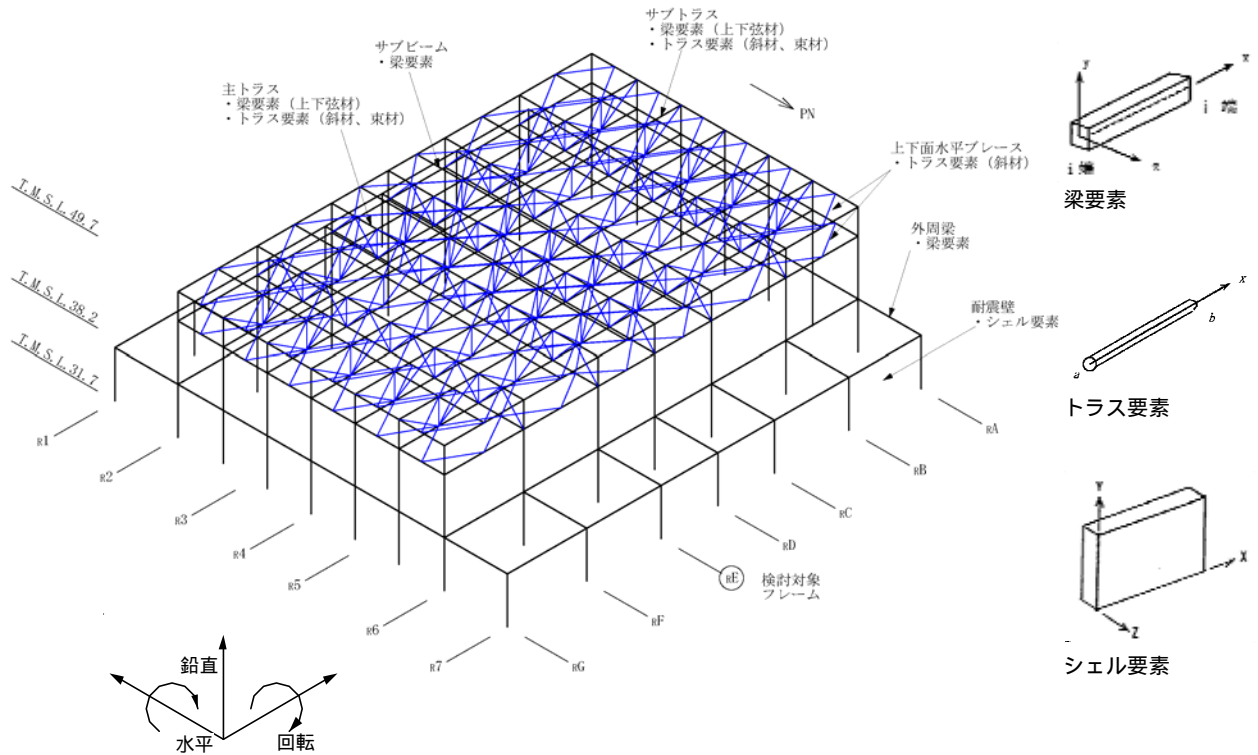
屋根トラスモデル化範囲
