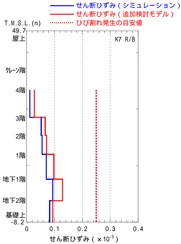
参図-12 RCCVの鉄筋コンクリート部のせん断ひずみ(南北方向)
