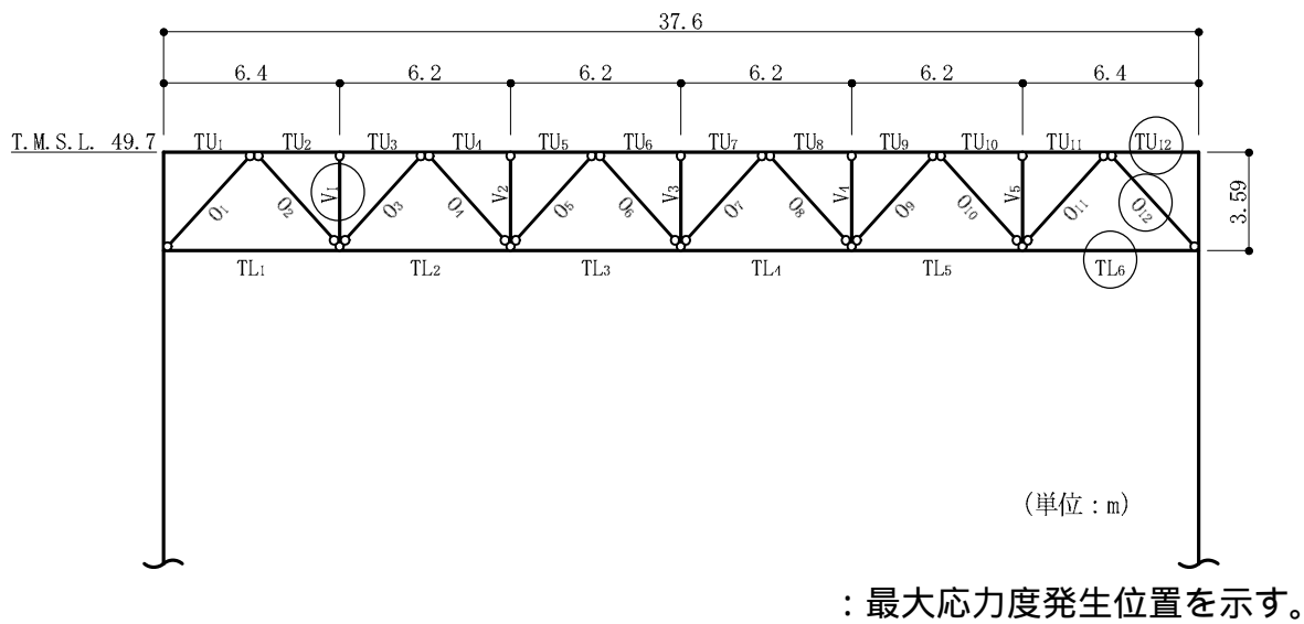
図-5.4.12 評価部位 ( R E 通り)
