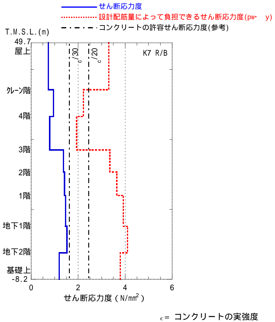
図-5.4.1 原子炉建屋 耐震壁のせん断応力度 (南北方向)
