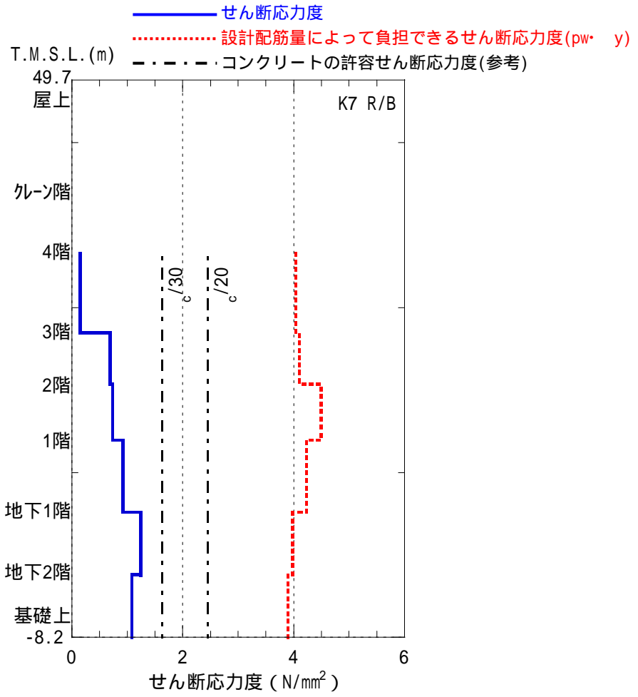
図-5.4.5 RCCVの鉄筋コンクリート部のせん断応力度 (南北方向)
