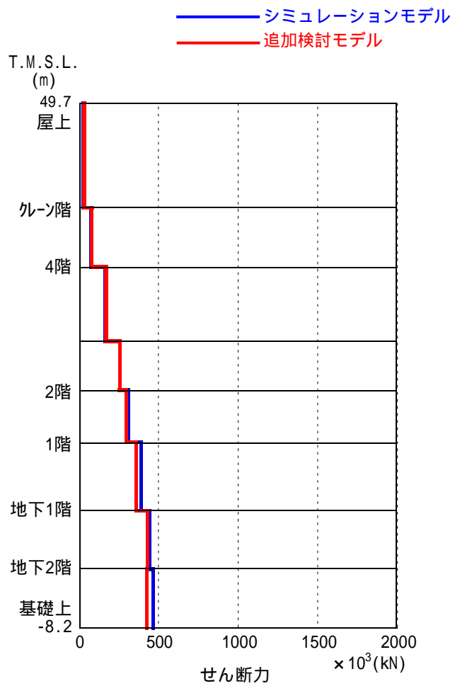
参図-14 原子炉建屋 最大応答せん断力 (南北方向)
