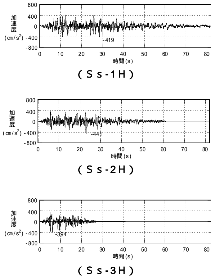
図5-4 加速度時刻歴波形 ( N S 方向 )
