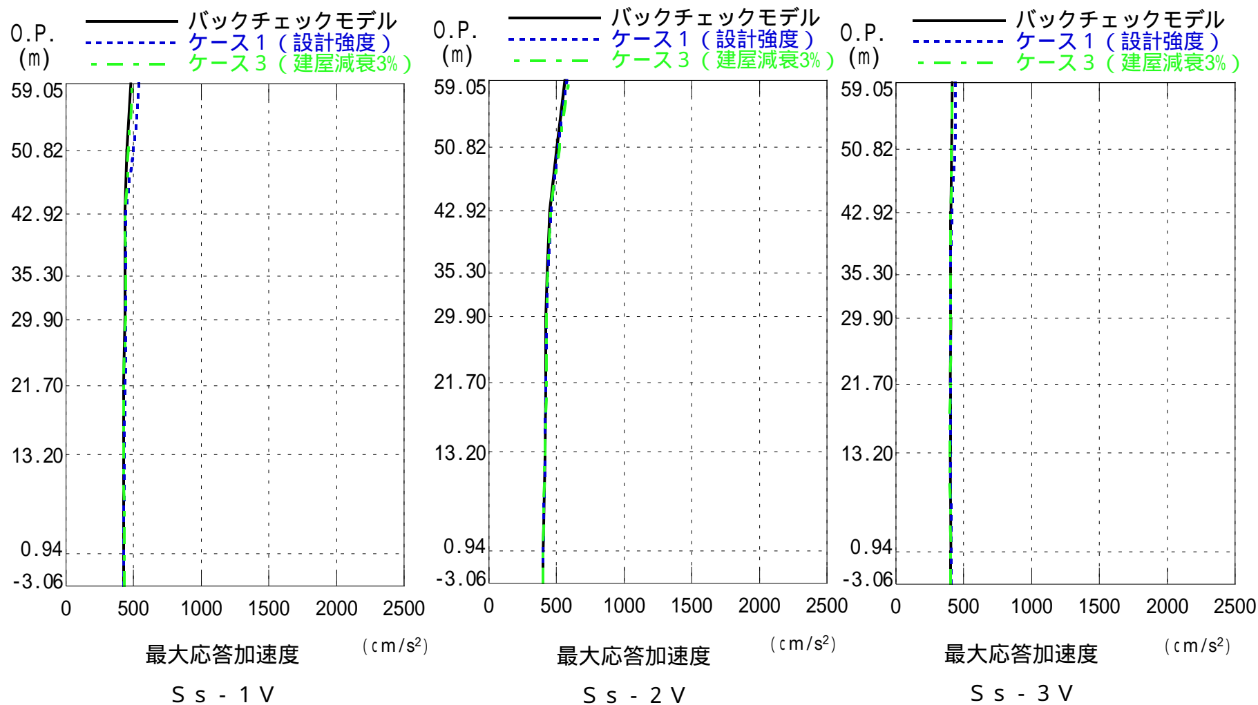
図4-7 最大応答加速度分布（鉛直方向）
