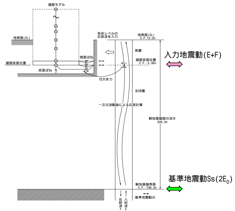
図5-1 基準地震動 S s から地震応答解析に至る評価フロー(水平方向)
