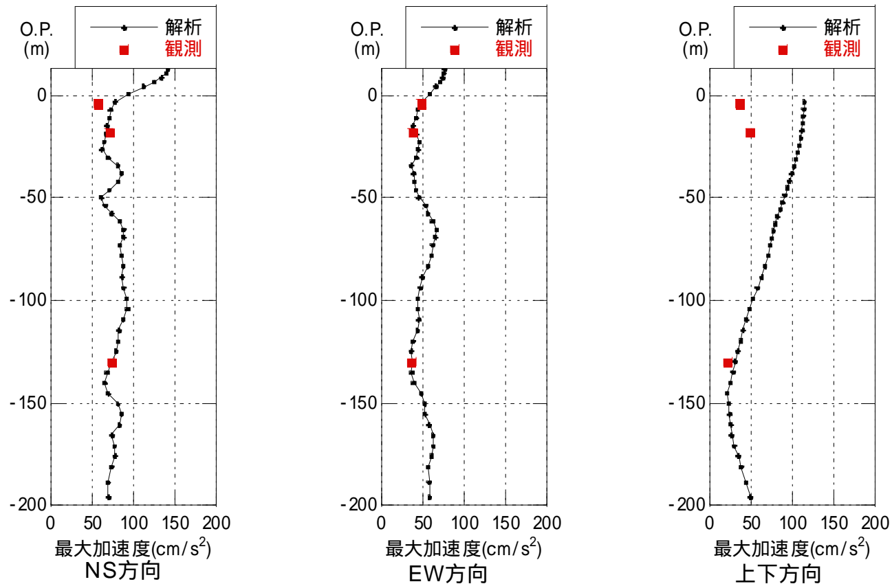
図3-4 地盤の最大応答加速度分布
