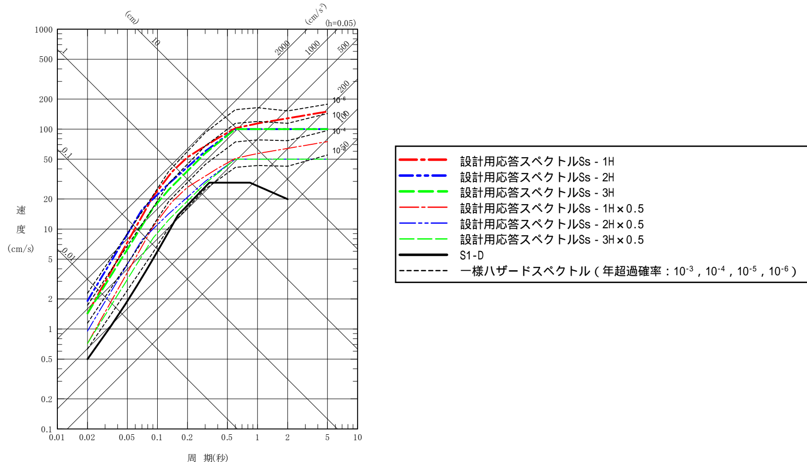
参図 - 1 弾性設計用地震動 S d の年超過確率
