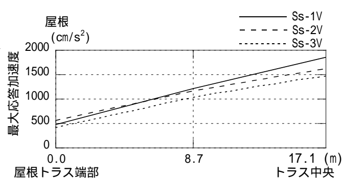
図5-22 最大応答加速度 (鉛直方向：屋根トラス)
