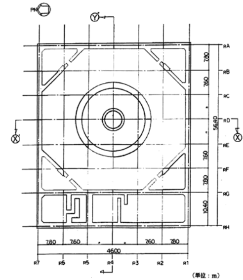
図1-2 平面図
