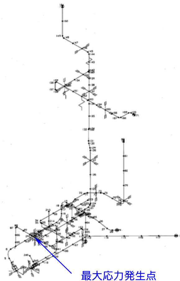
残留熱除去系配管
