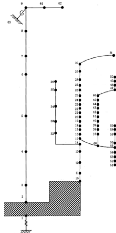
炉内構造物のモデル化（鉛直方向）
