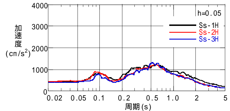
図5-5 入力地震動の応答スペクトル ( 基礎底面E+F/N S 方向 )
