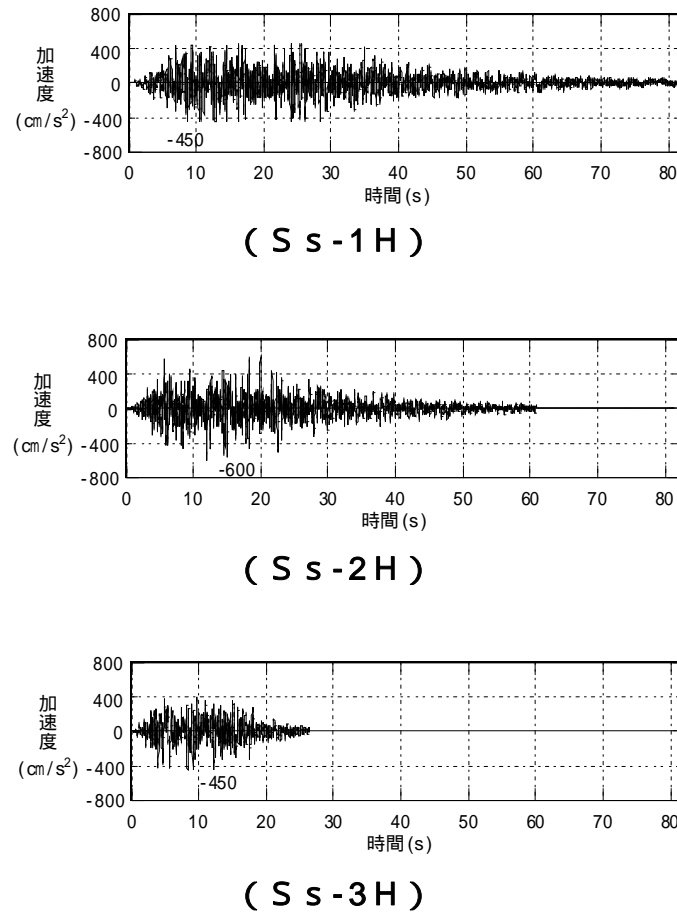
図5-2 加速度時刻歴波形 ( N S 方向 )
