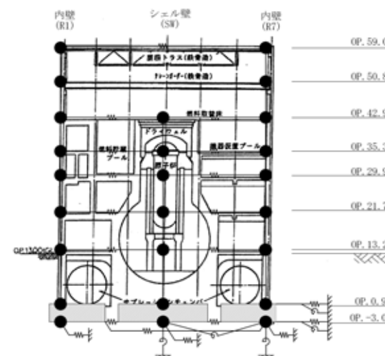
図4-11 床柔モデル (EW方向)
