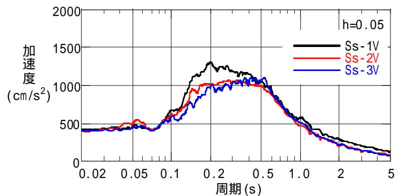
図5-14 床応答スペクトル (O.P.0.94m/鉛直方向)
