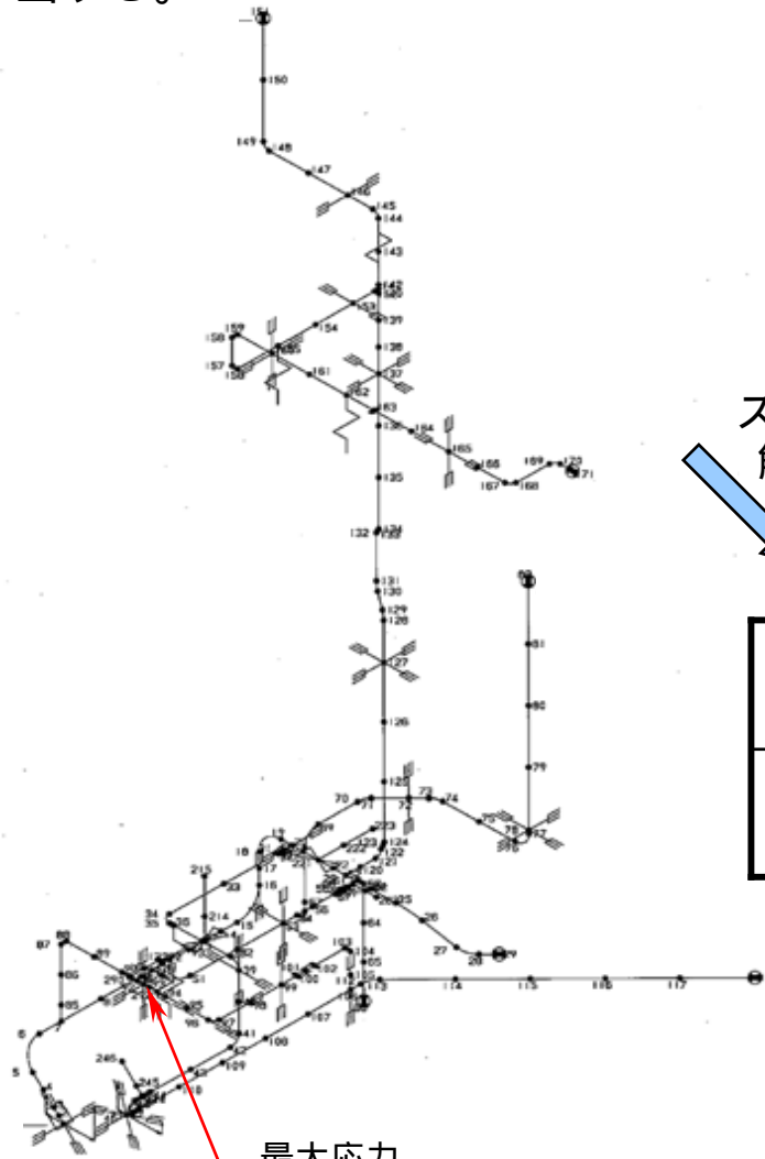
最大応力 発生点
