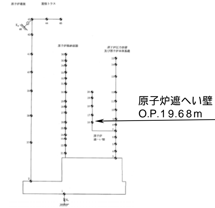
PCV-RPV鉛直方向解析モデル
