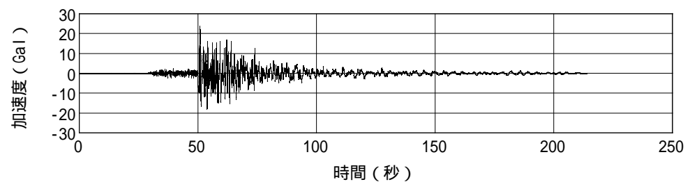
図4-14 加速度時刻歴波形 EW方向 Max=24 Gal
