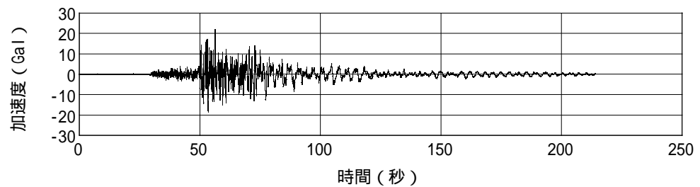
図4-13 加速度時刻歴波形 NS方向 Max=22 Gal
