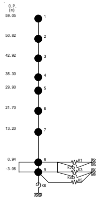
原子炉建屋解析モデル
