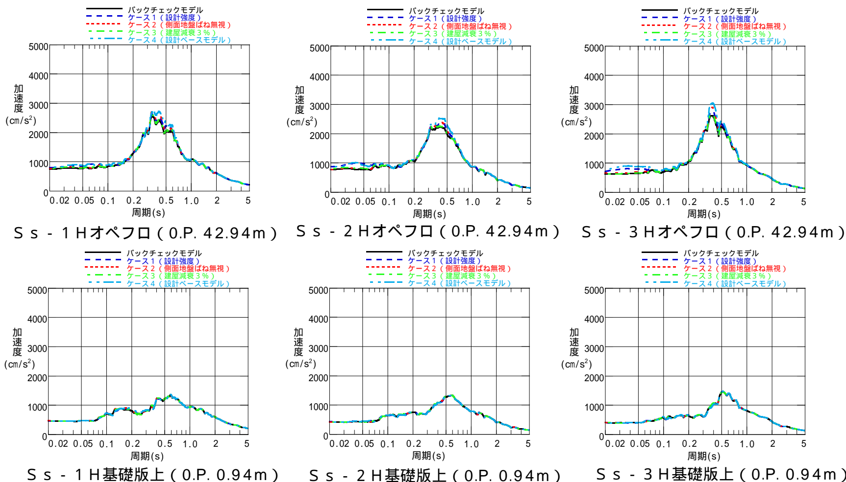
図4-6 床応答スペクトル（EW方向：h=0.05）
