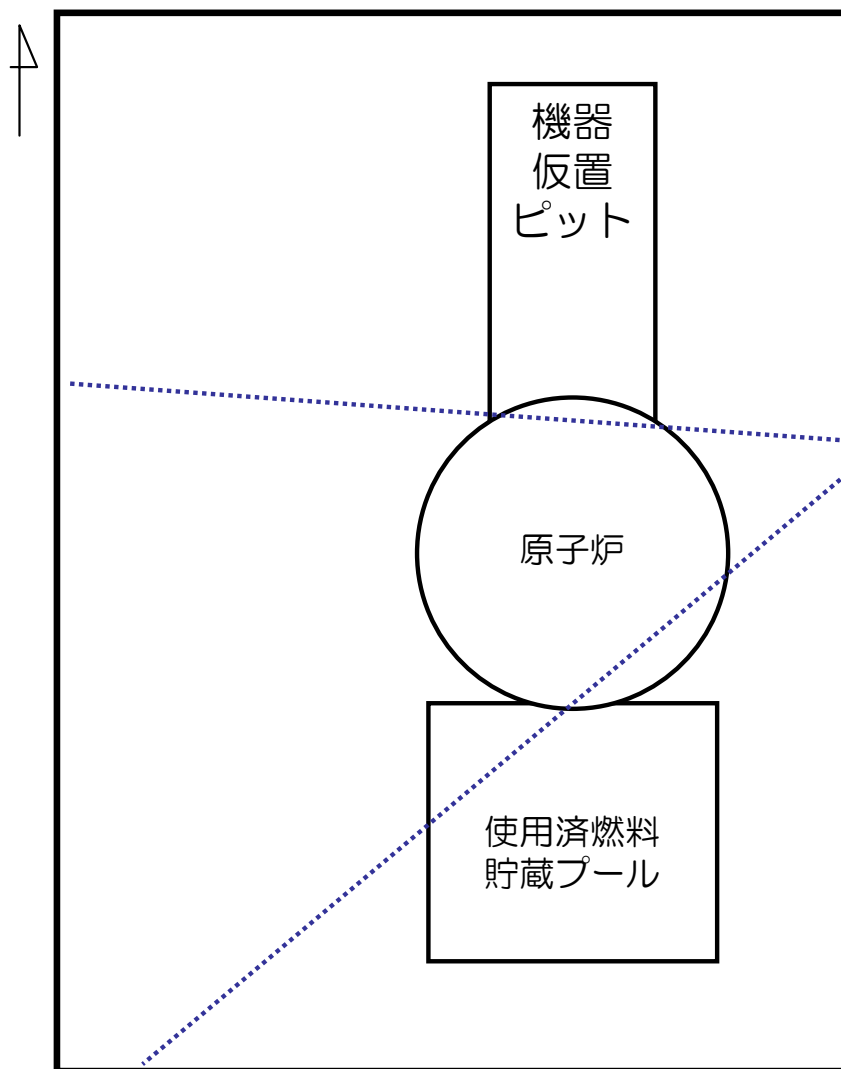
福島第一原子力発電所2号機原子炉建屋5階配置図
