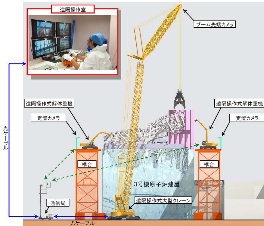
図1 福島第一原子力発電所3号機 原子炉建屋上部の瓦礫撤去イメージ
