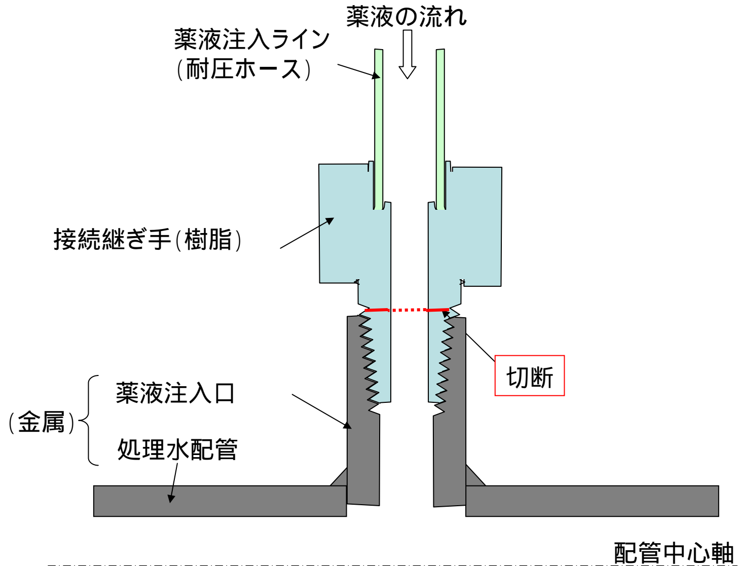
凝集沈殿装置薬液注入ライン損傷部の概略構造
