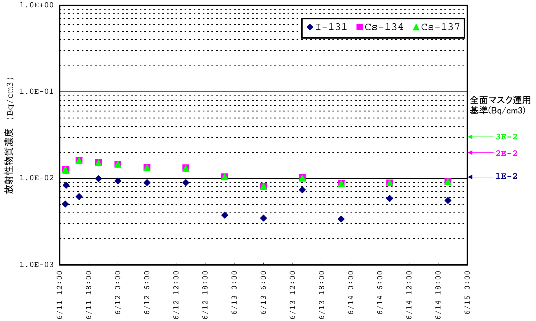
福島第一原子力発電所2号機 原子炉建屋内空气中放射性物質濃度推移
