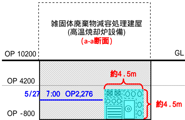
雑固体廃棄物減容処理建屋位置関係図
