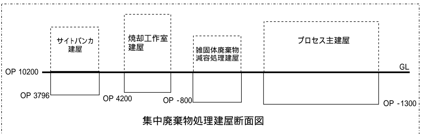
雑固体廃棄物減容処理建屋位置関係図
