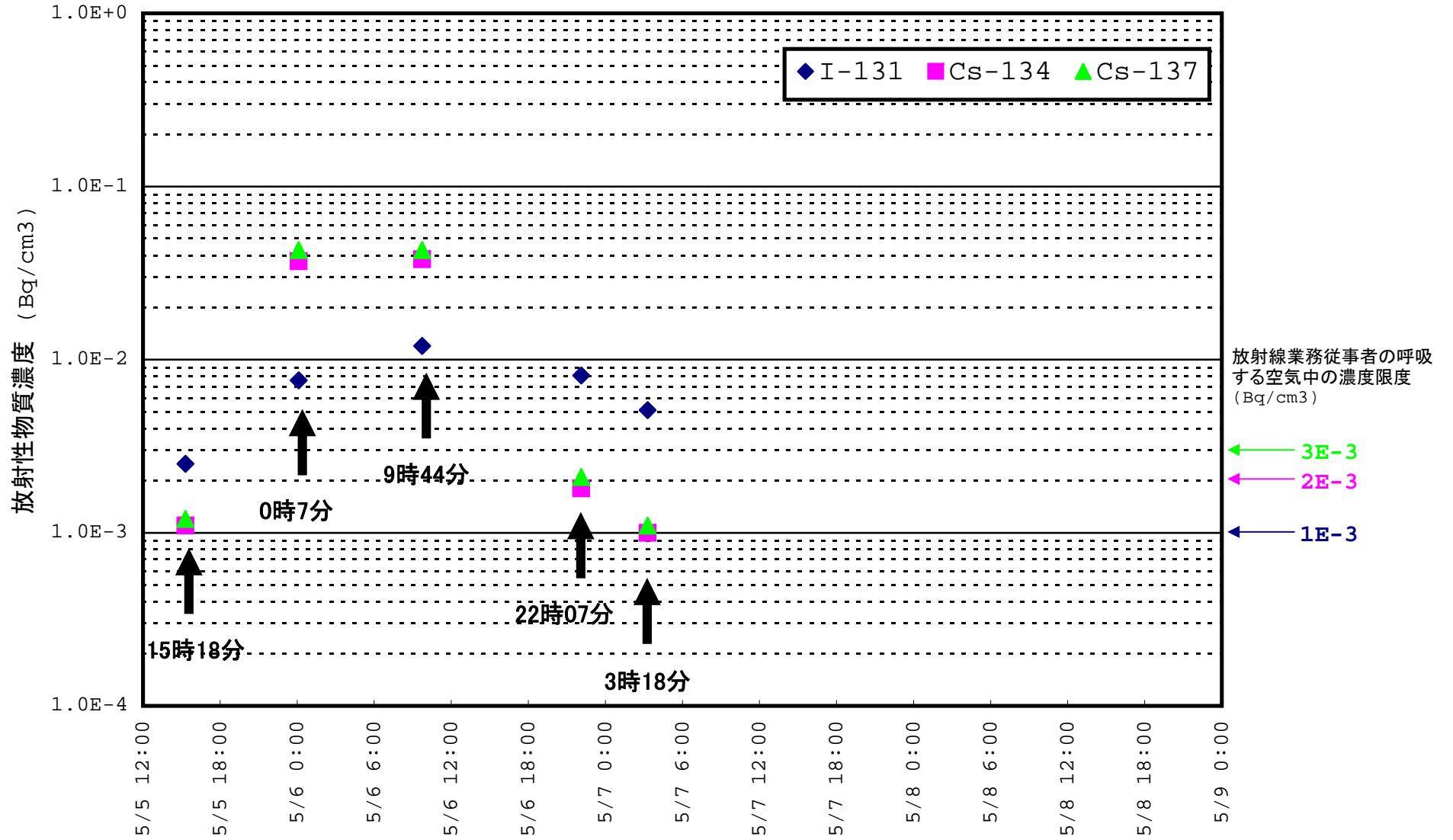
1号機 R/B内空气中放射性物質濃度推移
