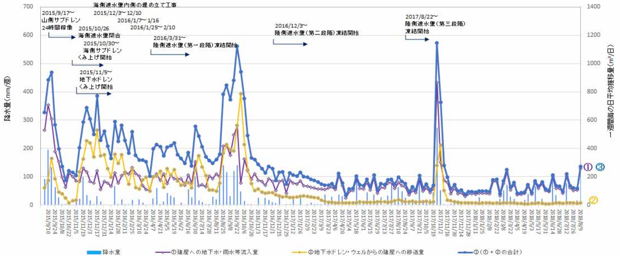
地下水ドレンからタービン建屋への移送量 ( 2018年8月2日 ~ 2018年8月8日 )
