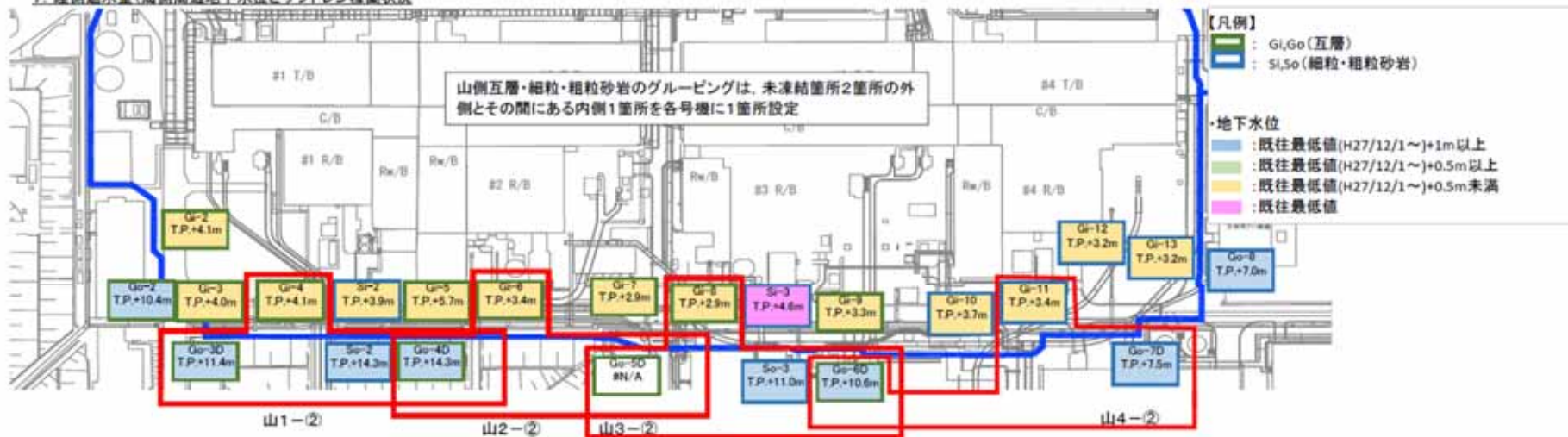
陸側遮水壁運用における監視項目(山側 互層、細粒・粗粒砂岩層水頭)
