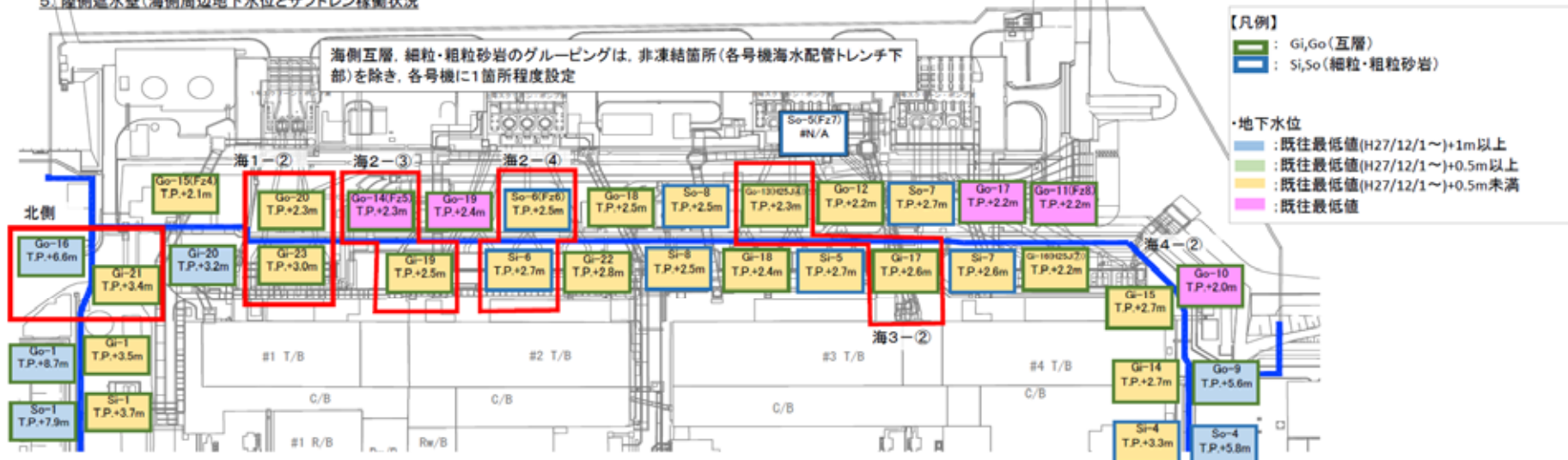
陸側遮水壁運用における監視項目(海側 互層、細粒・粗粒砂岩水位)
