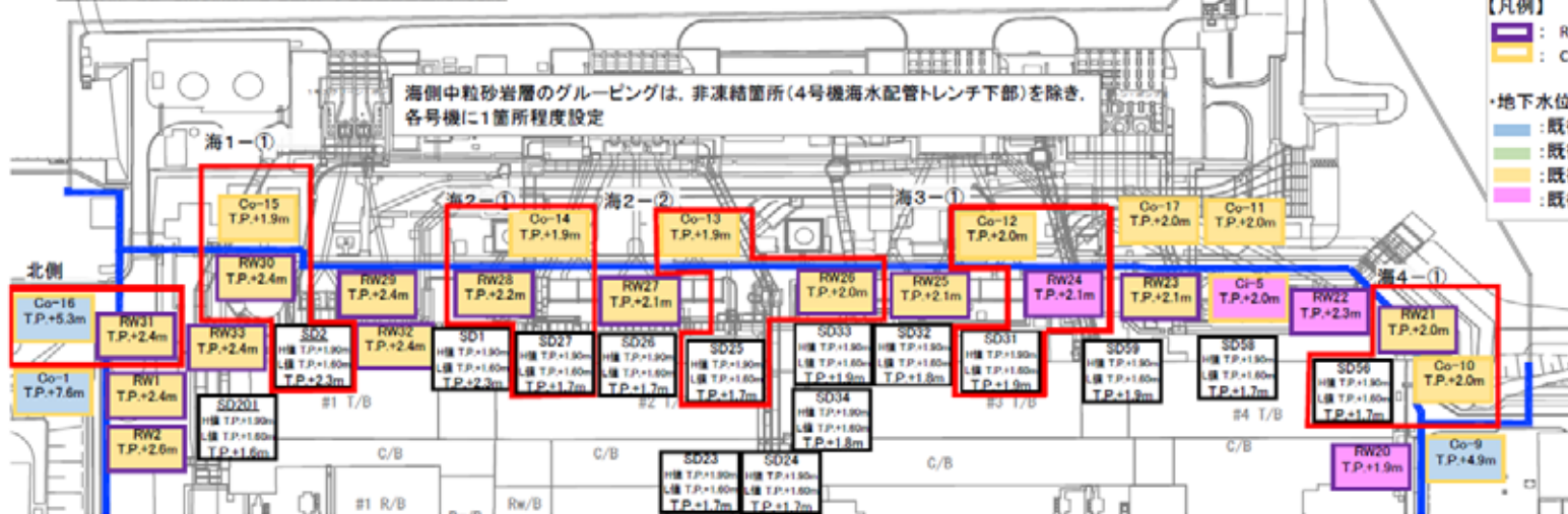
陸側遮水壁運用における監視項目(海側 中粒砂岩層水位)
