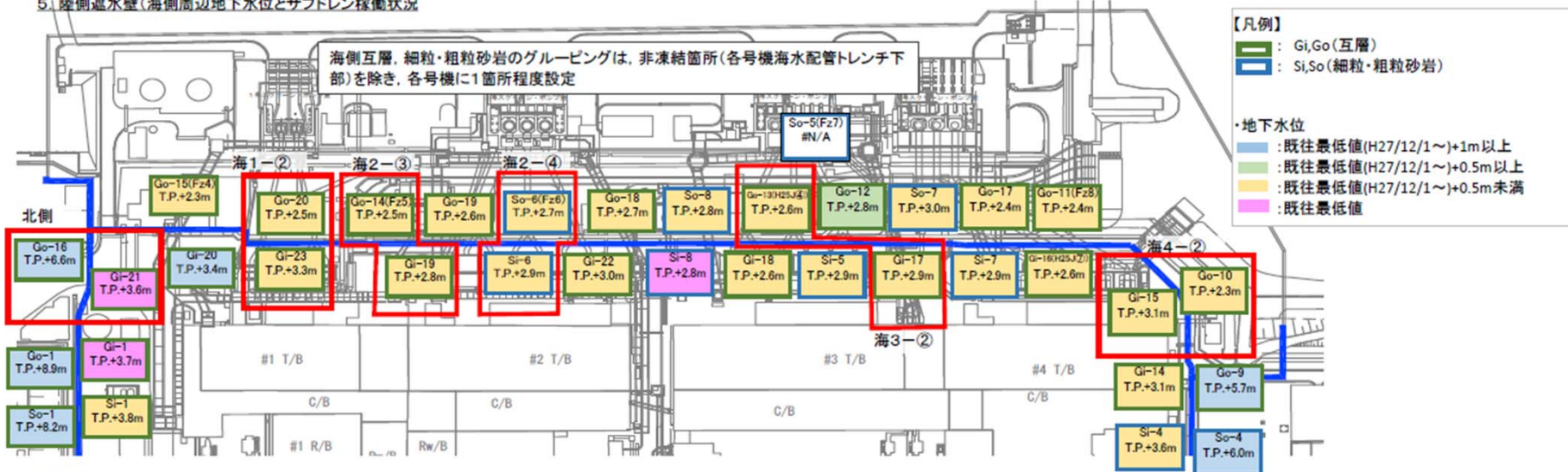
陸側遮水壁運用における監視項目（海側 互層、細粒・粗粒砂岩層水頭①）
