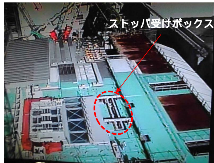
ストッパ受けボックス 吊り下ろし完了
