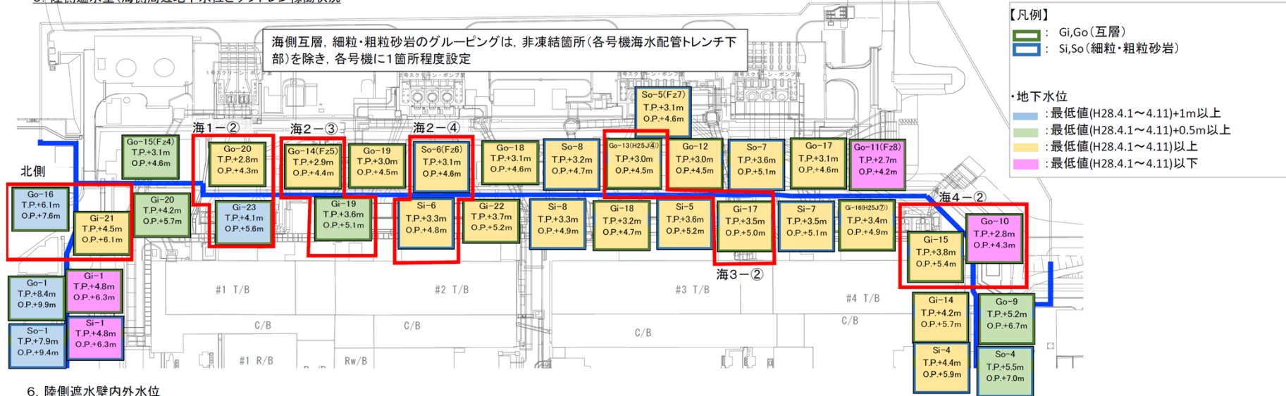
陸側遮水壁運用初期における監視項目（第一階段フェーズ2 海側 互層、細粒・粗粒砂岩水頭）
