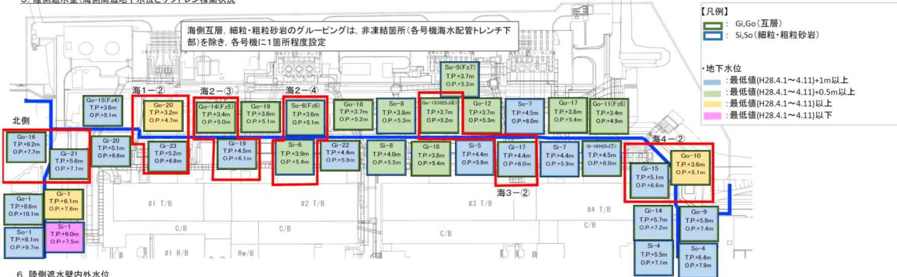
陸側遮水壁運用初期における監視項目（第一階段フェーズ2 海側 互層・細粒・粗粒砂岩水位）
