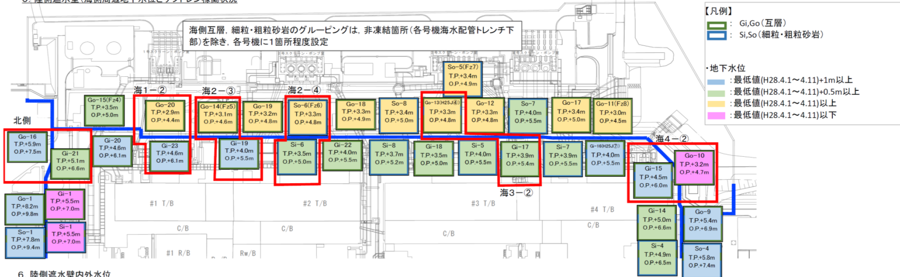
陸側遮水壁運用初期における監視項目（第一階段フェーズ2 海側 互層・細粒・粗粒砂岩水位）
