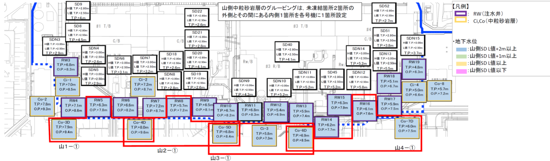
陸側遮水壁運用初期における監視項目(第一段階フェーズ2 山側 中粒砂岩層水位)
