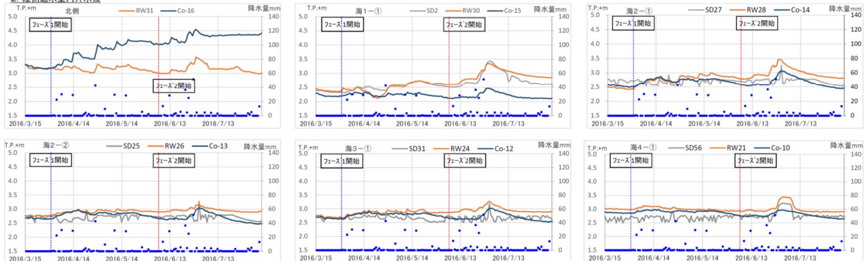
2. 陸側遮水壁内外水位
