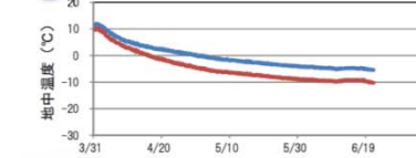
11 250-7S 中粒砂岩層 (5.9°C) ※凍土ラインと測温管 250-7S 互層部 (3.2°C) の距離 786mm
