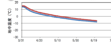
17 500-11S 中粒砂岩層 (-7.6°C) ※凍土ラインと測温管 500-11S 互層部 (-5.9°C) の距離 736mm
