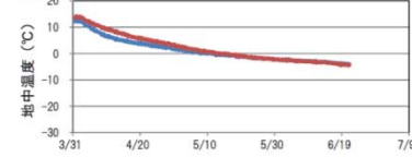
8 130-5S 中粒砂岩層 (-4°C) ※凍土ラインと測温管 130-5S 互層部 (-4.3°C) の距離 794mm
