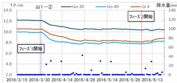
8. 陸側遮水壁内外水位
