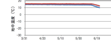
13 130-8S 中粒砂岩層 (-2.3°C) ※凍土ラインと測温管 130-8S 互層部 (-1.6°C) の距離 803mm
