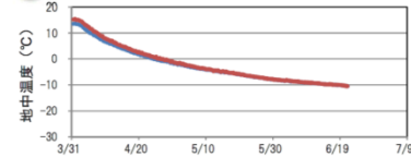
19 290-12S 中粒砂岩層 (-10.5°C) ※凍土ラインと測温管 290-12S 互層部 (-10.5°C) の距離 765mm
