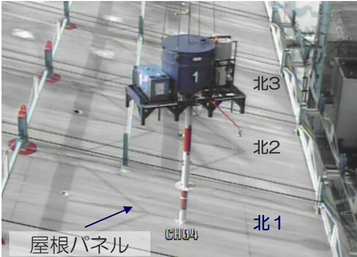
北1 屋根パネル飛散防止剤散布状況
